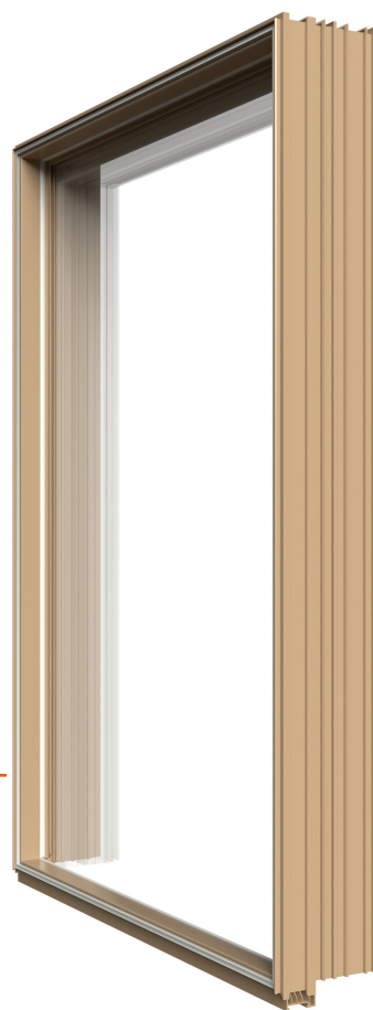
Controtelaio FIN-Fix prolungato per fissaggio persiana e attacco termoisolato bancale finestra
