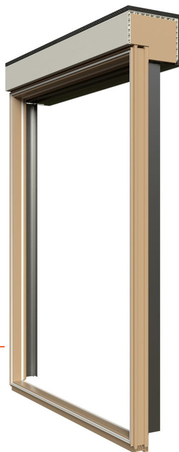
Controtelaio FIN-Fix con cassonetto per ombreggiante in tessuto e attacco termoisolato bancale finestra
