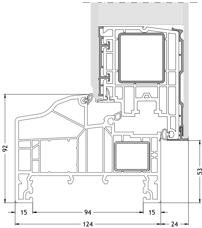
Dormant en L 951 ouverture vers l'intérieur avec ouvrant T926 Échelle 1:2
