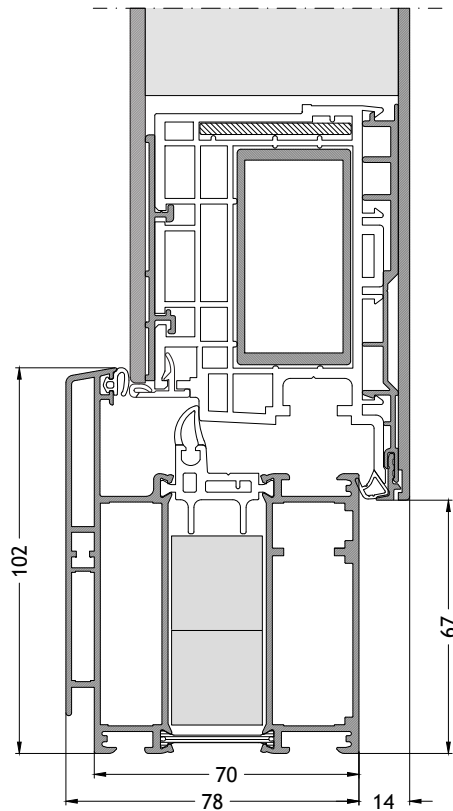
Dormant en L 711 ouverture vers l'intérieur avec ouvrant A96 Échelle 1:2
