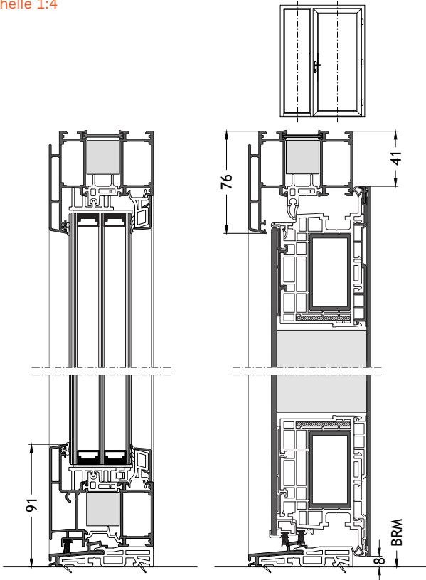
Seuil plat S0 ouverture vers l'intérieur avec ouvrant A96 Échelle 1:4
