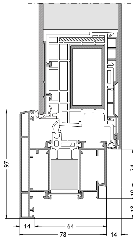
Dormant en Z/T 718 ouverture vers l'intérieur avec ouvrant A96 Échelle 1:2
