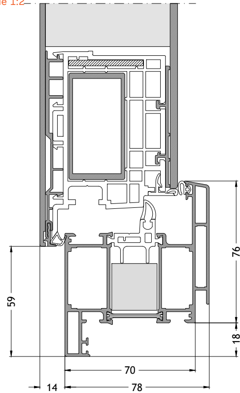
Dormant en L A712 ouverture vers l'extérieur avec ouvrant A96A Échelle 1:2
