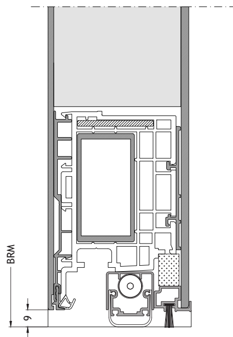
Seuil plat A4 ouverture vers l'extérieur avec ouvrant A96A Échelle 1:2
