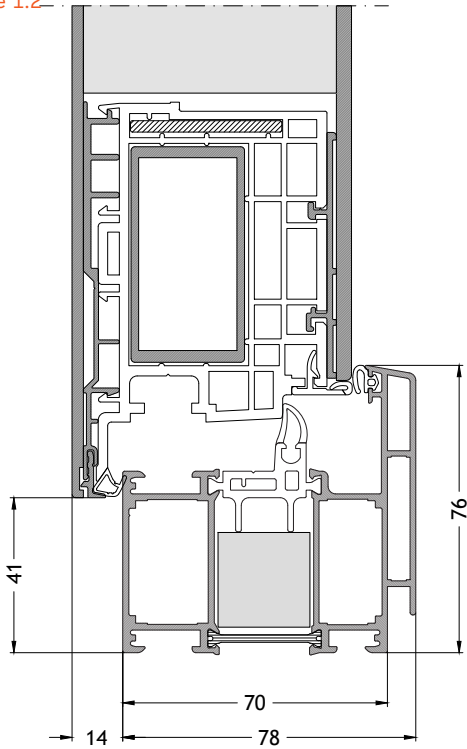
Dormant en L A705 ouverture vers l'extérieur avec ouvrant A96A Échelle 1:2
