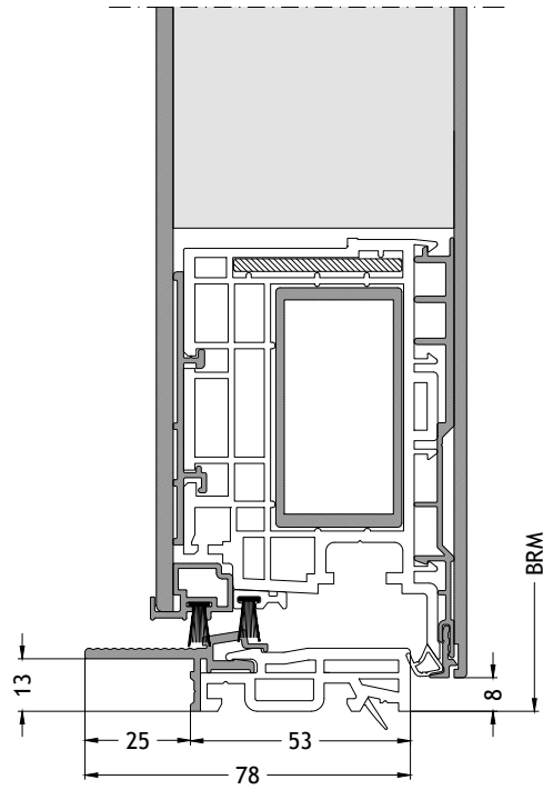
Seuil plat S2 ouverture vers l'intérieur avec ouvrant A96 Échelle 1:2
