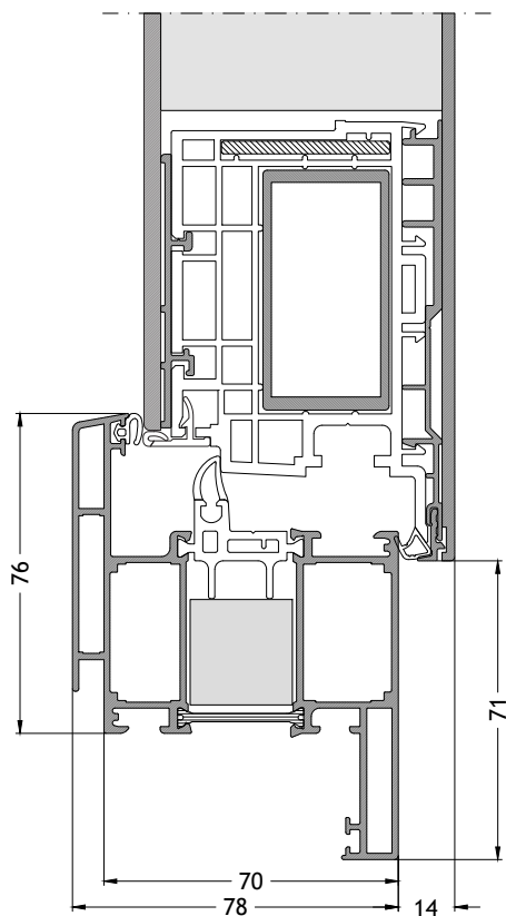
Dormant en Z 719 ouverture vers l'intérieur avec ouvrant A96 Échelle 1:2
