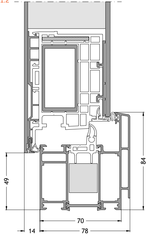
Dormant en L A706 ouverture vers l'extérieur avec ouvrant A96A Échelle 1:2
