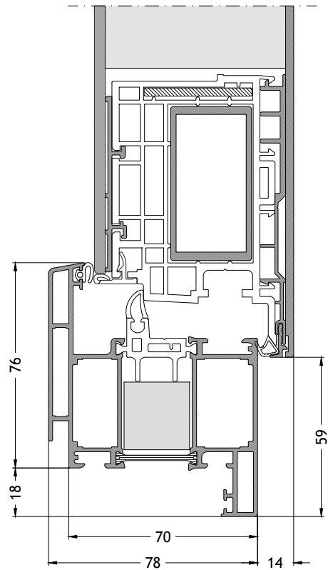
Dormant en Z/T 712 ouverture vers l'intérieur avec ouvrant A96 Échelle 1:2
