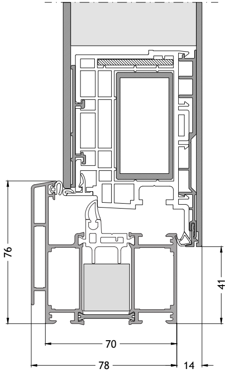
Dormant en L 705 ouverture vers l'intérieur avec ouvrant A96 Échelle 1:2
