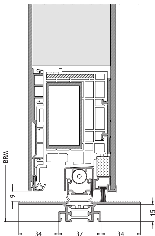
Seuil plat A3 ouverture vers l'extérieur avec ouvrant A96A Échelle 1:2
