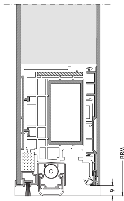
Seuil plat S4 ouverture vers l'intérieur avec ouvrant A96 Échelle 1:2
