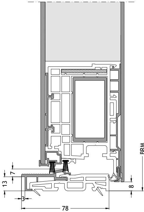
Seuil plat S1 ouverture vers l'intérieur avec ouvrant A96 Échelle 1:2
