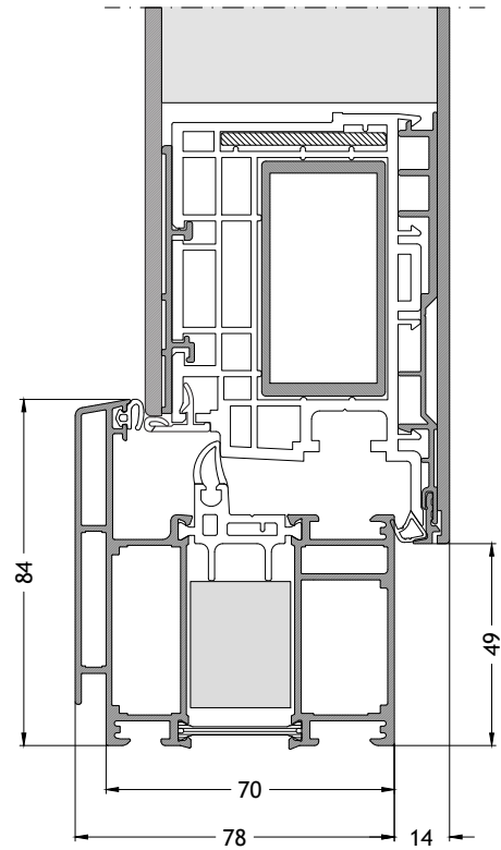
Dormant en L 706 ouverture vers l'intérieur avec ouvrant A96 Échelle 1:2
