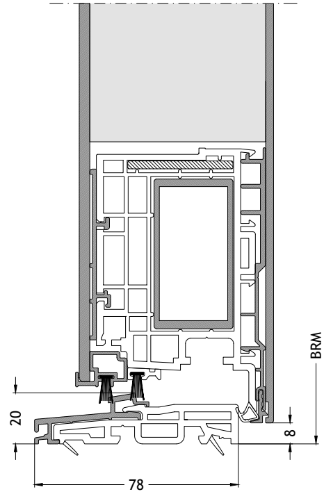
Seuil plat S0 ouverture vers l'intérieur avec ouvrant A96 Échelle 1:2
