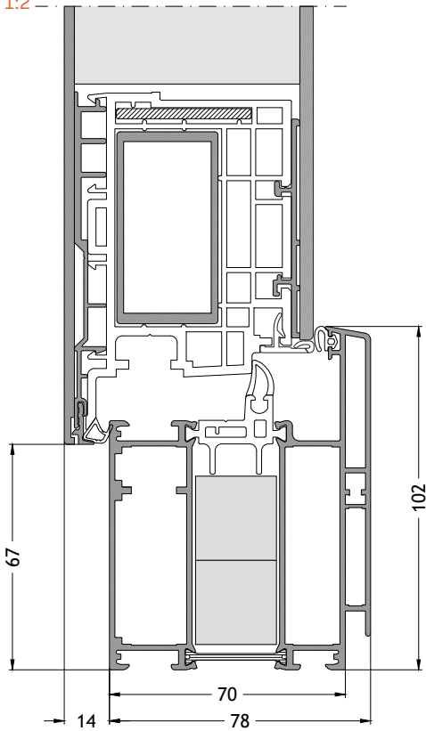
Dormant en L A711 ouverture vers l'extérieur avec ouvrant A96A Échelle 1:2
