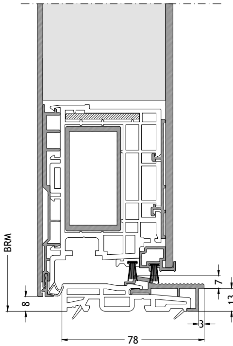
Seuil plat A1 ouverture vers l'extérieur avec ouvrant A96A Échelle 1:2
