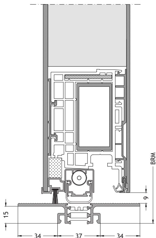
Seuil plat S3 ouverture vers l'intérieur avec ouvrant A96 Échelle 1:2
