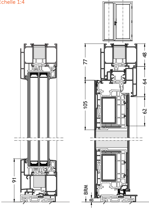
Seuil plat A1 ouverture vers l'extérieur avec ouvrant A96A Échelle 1:4
