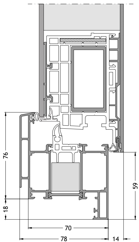
Telaio forma a Z/T 712 apertura verso l'interno con anta A96 Scala 1:2
