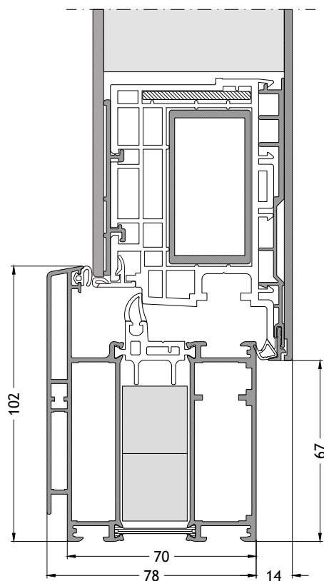
Telaio forma ad L 711 apertura verso l'interno con anta A96 Scala 1:2
