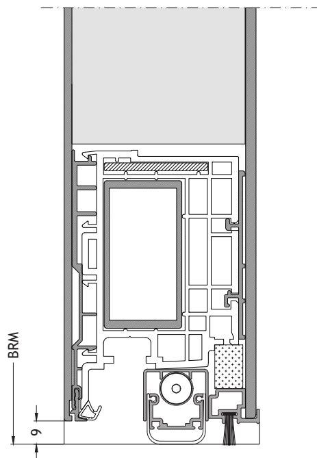
Soglia ribassata A4 apertura verso l'esterno con anta A96A Scala 1:2
