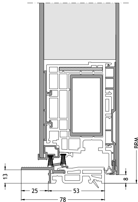
Soglia ribassata S2 apertura verso l'interno con anta A96
