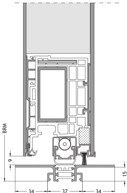
Soglia ribassata A3 apertura verso l'esterno con anta A96A Scala 1:2
