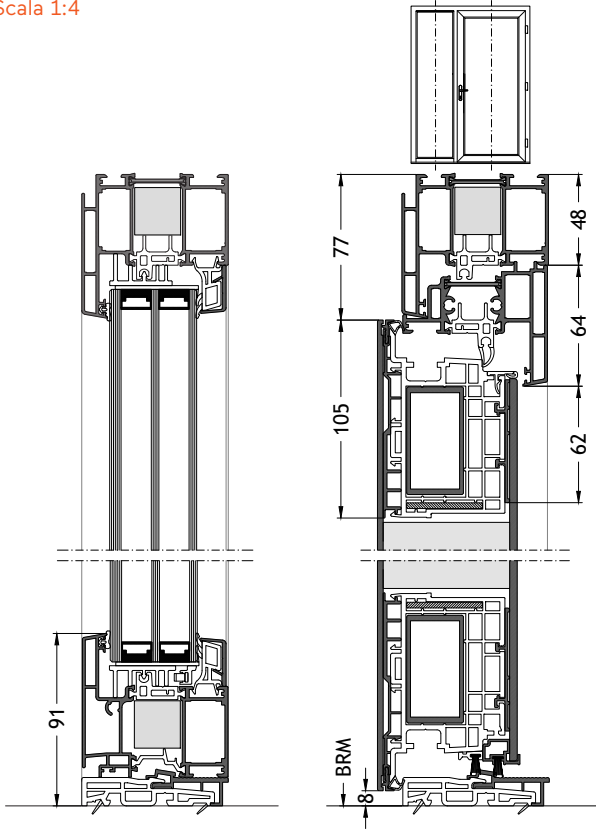
Soglia ribassata A1 apertura verso l'esterno con anta A96A Scala 1:4
