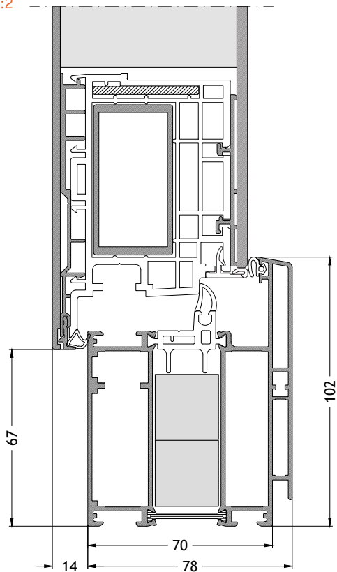
Telaio forma ad L A711 apertura verso l'esterno con anta A96A Scala 1:2
