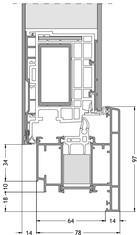
Telaio forma ad L A718 apertura verso l'esterno con anta A96A
