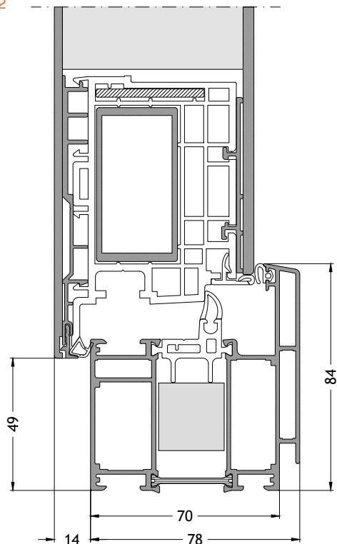
Telaio forma ad L A706 apertura verso l'esterno con anta A96A Scala 1:2
