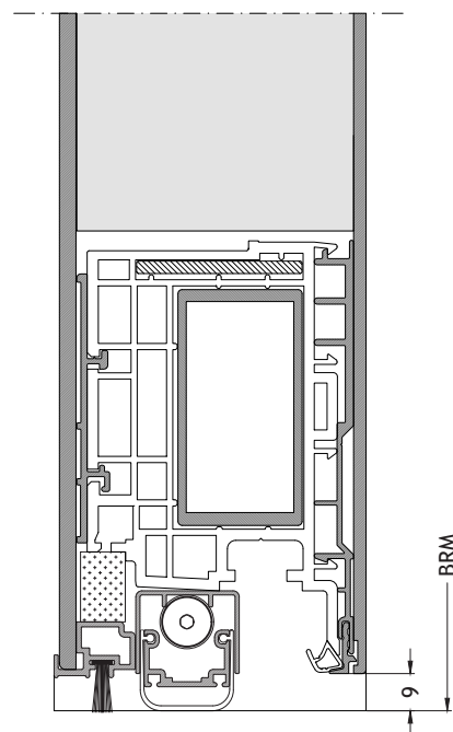
Soglia ribassata S4 apertura verso l'interno con anta A96 Scala 1:2
