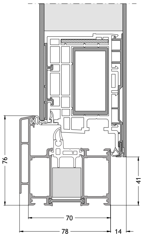
Telaio forma ad L 705 apertura verso l'interno con anta A96 Scala 1:2
