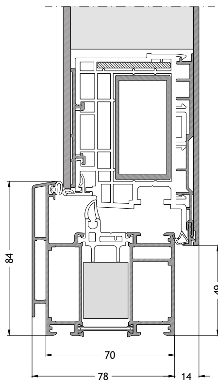
Telaio forma ad L 706 apertura verso l'interno con anta A96 Scala 1:2
