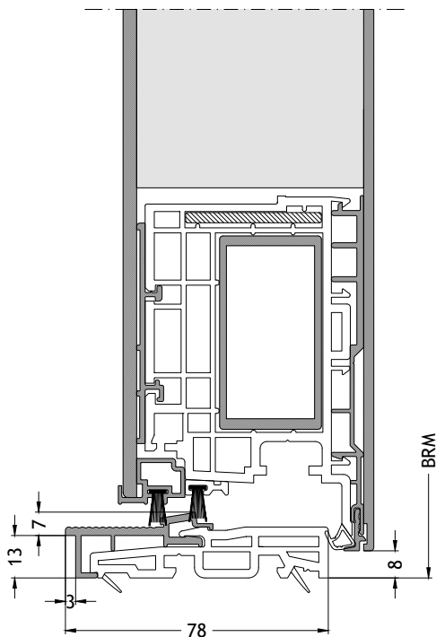
Soglia ribassata S1 apertura verso l'interno con anta A96
