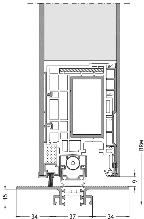
Soglia ribassata S3 apertura verso l'interno con anta A96 Scala 1:2
