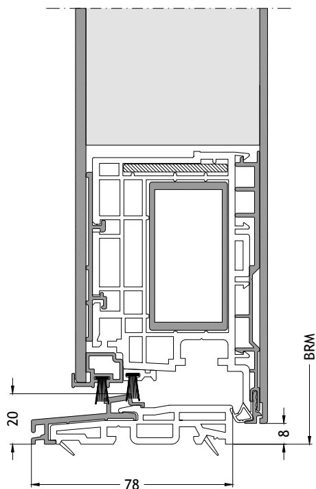
Soglia ribassata S0 apertura verso l'interno con anta A96
