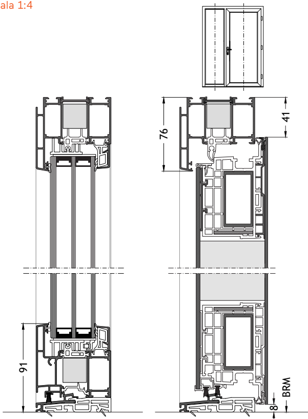
Soglia ribassata S0 apertura verso l'interno con anta A96
