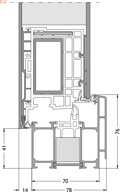
Telaio forma ad L A705 apertura verso l'esterno con anta A96A Scala 1:2
