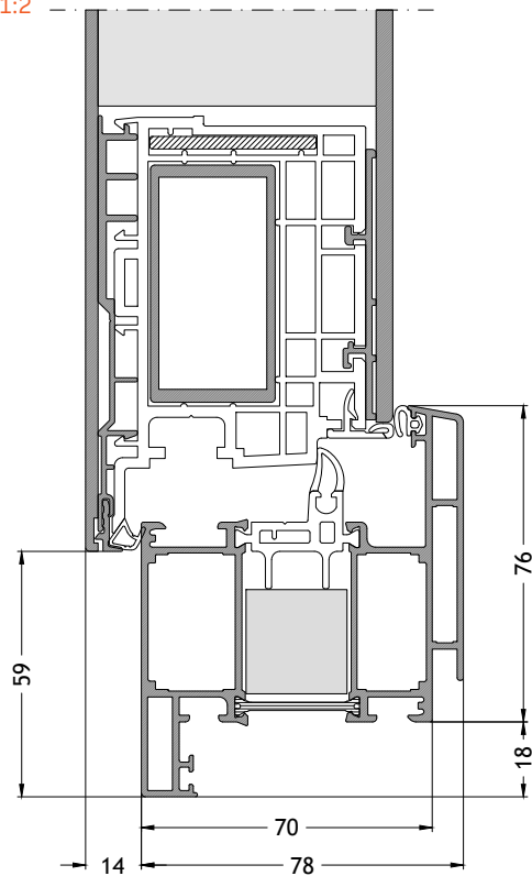
Telaio forma ad L A712 apertura verso l'esterno con anta A96A Scala 1:2
