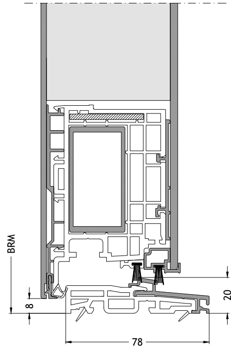
Soglia ribassata A0 apertura verso l'esterno con anta A96A Scala 1:2
