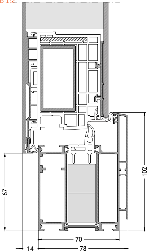
Blendrahmen L-Form A711 nach außen öffnend mit Flügel A96A Maßstab 1:2
