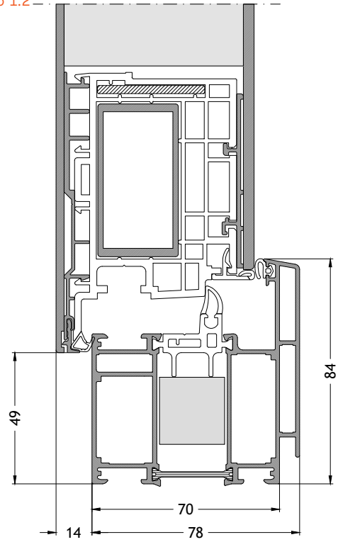
Blendrahmen L-Form A706 nach außen öffnend mit Flügel A96A Maßstab 1:2
