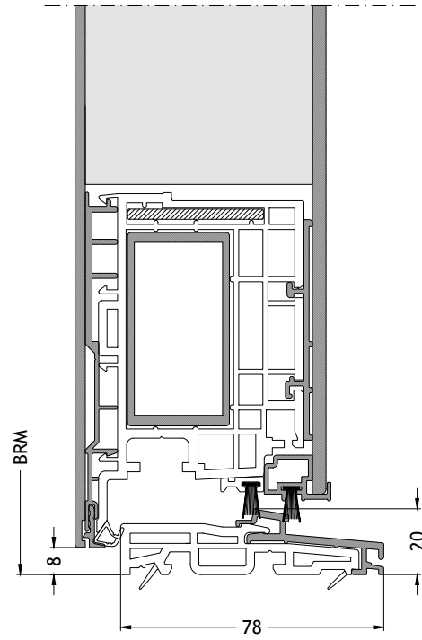
Flache Bodenschwelle A0 nach außen öffnend mit Flügel A96A Maßstab 1:2
