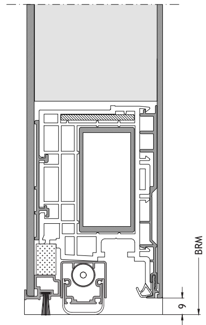
Flache Schwelle S4 nach innen öffnend mit Flügel A96 Maßstab 1:2
