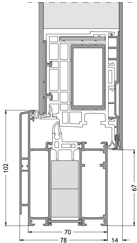
Blendrahmen L-Form 711 nach innen öffnend mit Flügel A96 Maßstab 1:2
