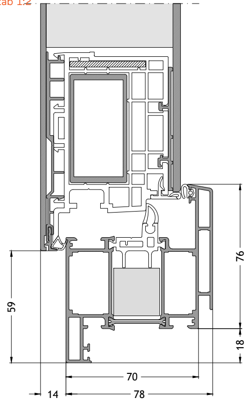
Blendrahmen L-Form A712 nach außen öffnend mit Flügel A96A Maßstab 1:2
