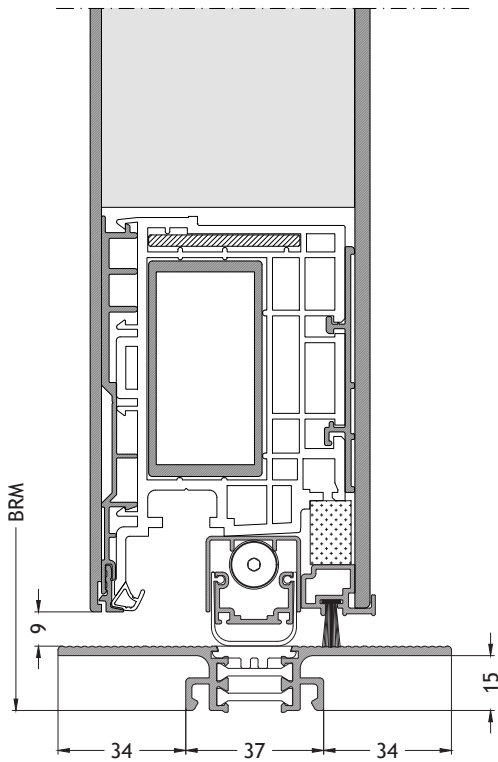
Flache Schwelle A3 nach außen öffnend mit Flügel A96A Maßstab 1:2
