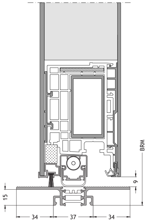
Flache Schwelle S3 nach innen öffnend mit Flügel A96 Maßstab 1:2
