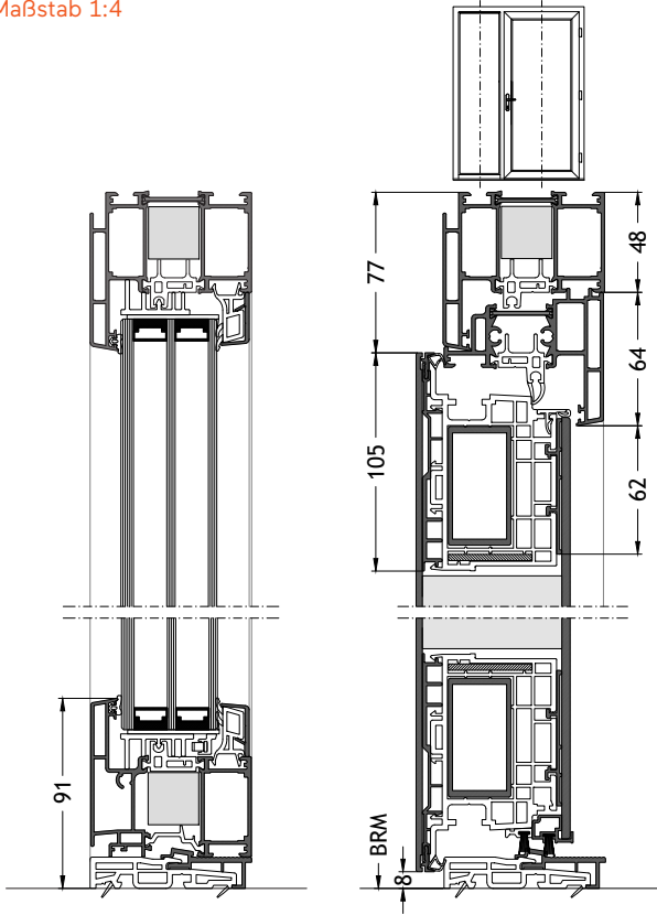
Flache Schwelle A1 nach außen öffnend mit Flügel A96A Maßstab 1:4
