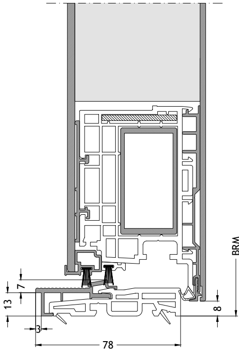
Flache Schwelle S1 nach innen öffnend mit Flügel A96 Maßstab 1:2
