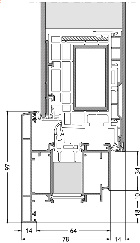
Blendrahmen Z-/T-Form 718 nach innen öffnend mit Flügel A96 Maßstab 1:2
