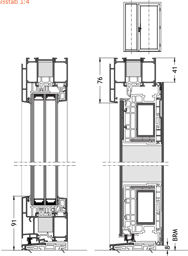
Flache Bodenschwelle S0 nach innen öffnend mit Flügel A96 Maßstab 1:4
