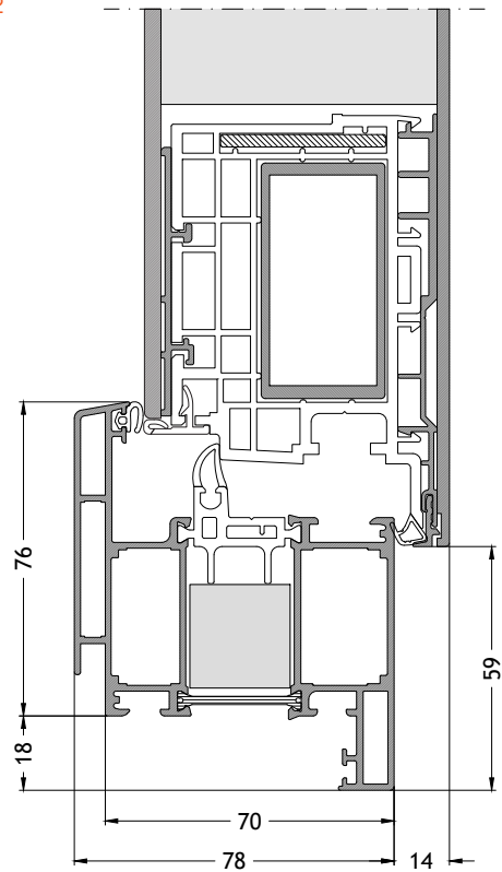
Blendrahmen Z-/T-Form 712 nach innen öffnend mit Flügel A96 Maßstab 1:2
