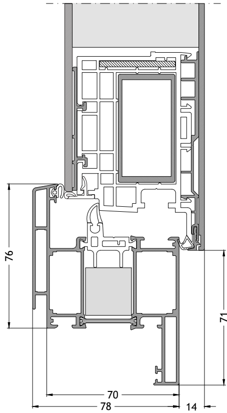
Blendrahmen Z-Form 719 nach innen öffnend mit Flügel A96 Maßstab 1:2
