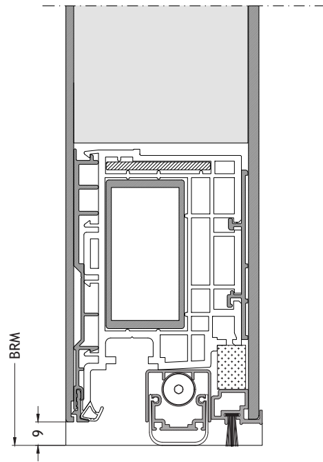
Flache Schwelle A4 nach außen öffnend mit Flügel A96A Maßstab 1:2
