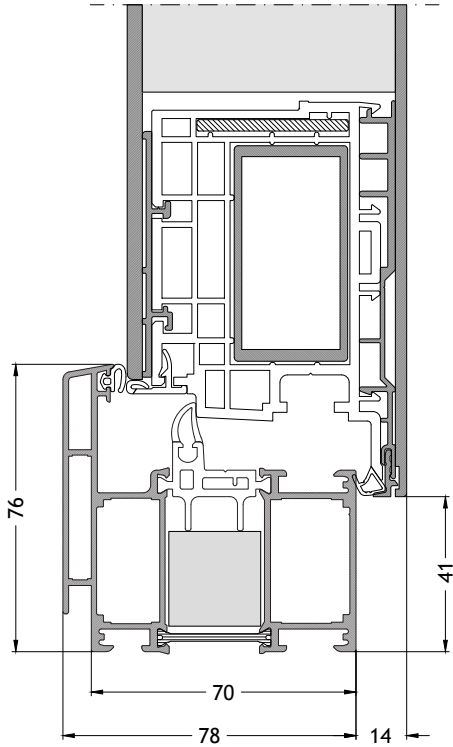
Blendrahmen L-Form 705 nach innen öffnend mit Flügel A96 Maßstab 1:2
