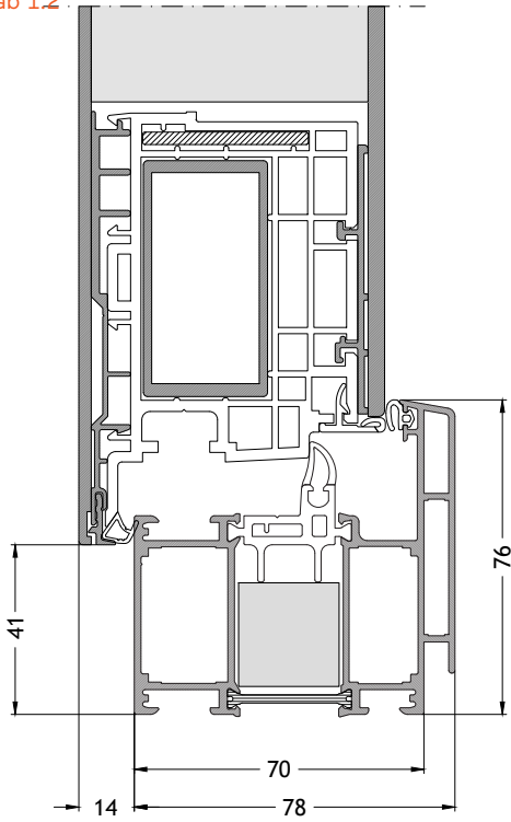
Blendrahmen L-Form A705 nach außen öffnend mit Flügel A96A Maßstab 1:2
