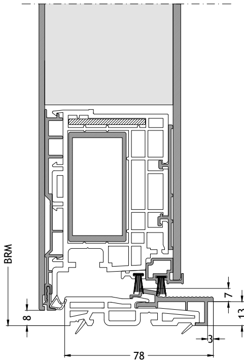
Flache Schwelle A1 nach außen öffnend mit Flügel A96A Maßstab 1:2
