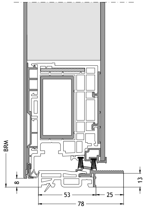
Flache Schwelle A2 nach außen öffnend mit Flügel A96A Maßstab 1:2
