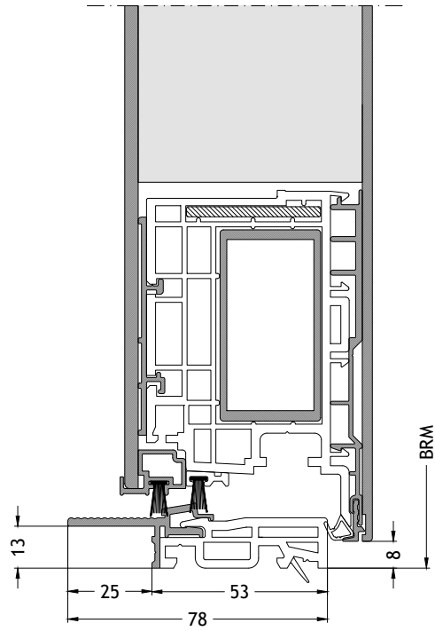
Flache Schwelle S2 nach innen öffnend mit Flügel A96 Maßstab 1:2
