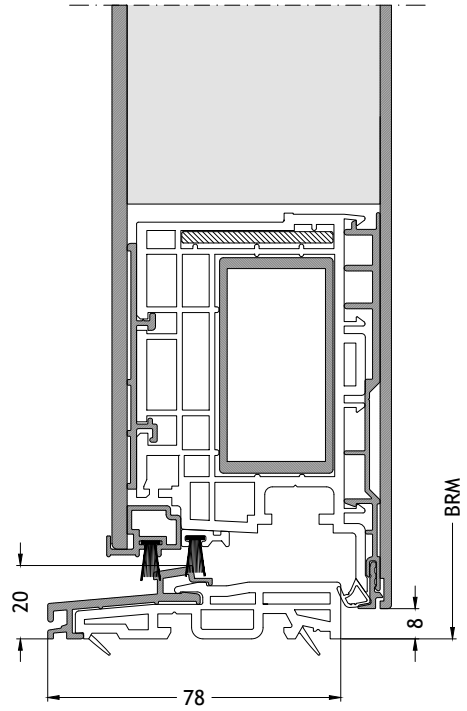
Flache Bodenschwelle S0 nach innen öffnend mit Flügel A96 Maßstab 1:2
