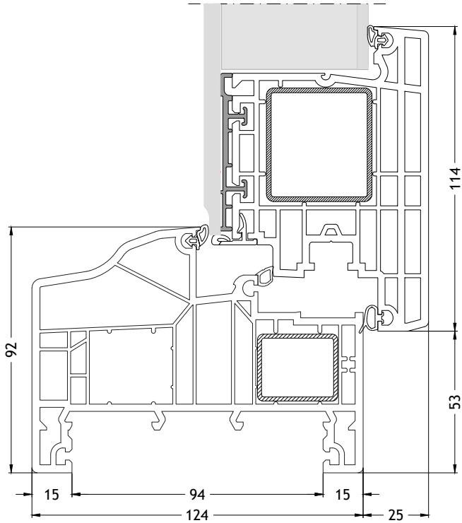
Dormant en L 951 ouverture vers l'intérieur avec ouvrant T936 Échelle 1:2
