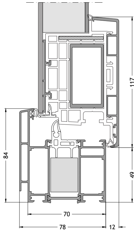
Dormant en L 706 ouverture vers l'intérieur avec ouvrant A95 Échelle 1:2
