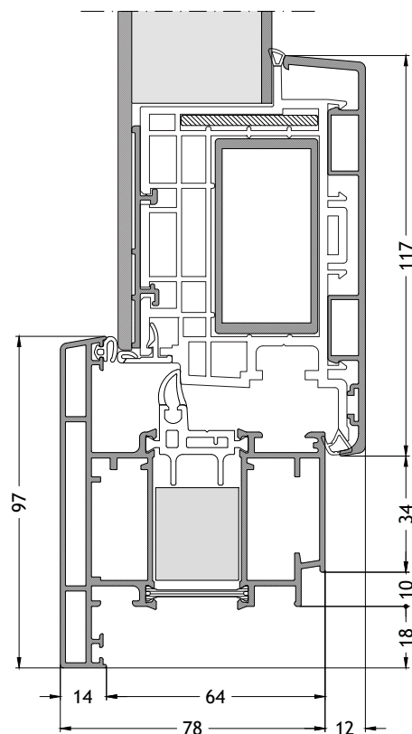
Dormant en Z/T 718 ouverture vers l'intérieur avec ouvrant A95 Échelle 1:2
