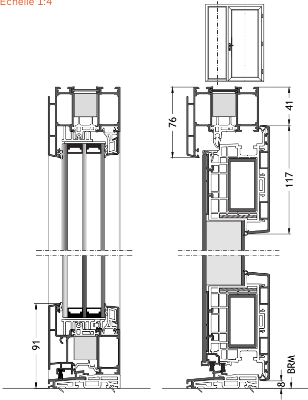
Seuil plat S0 ouverture vers l'intérieur avec ouvrant A95 Échelle 1:4
