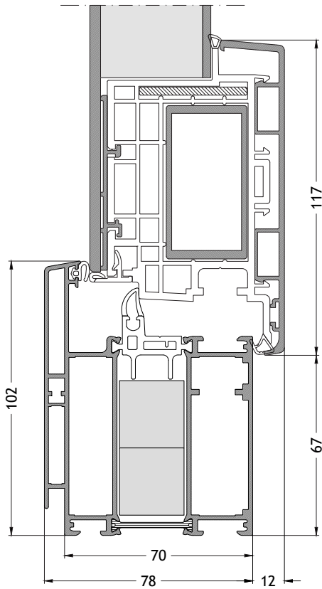
Dormant en L 711 ouverture vers l'intérieur avec ouvrant A95 Échelle 1:2
