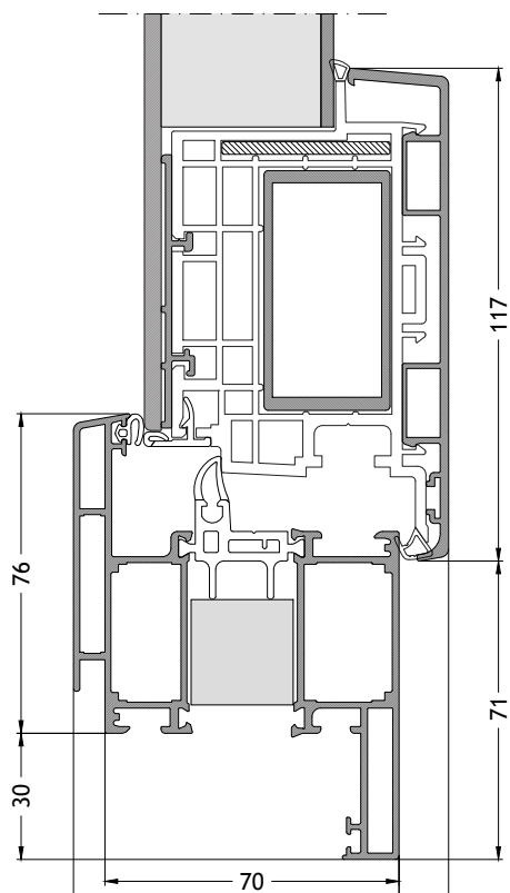
Dormant en Z 719 ouverture vers l'intérieur avec ouvrant A95 Échelle 1:2
