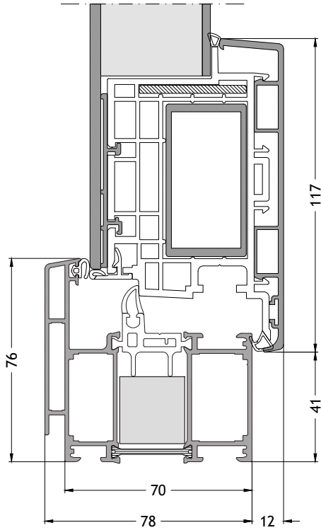
Dormant en L 705 ouverture vers l'intérieur avec ouvrant A95 Échelle 1:2
