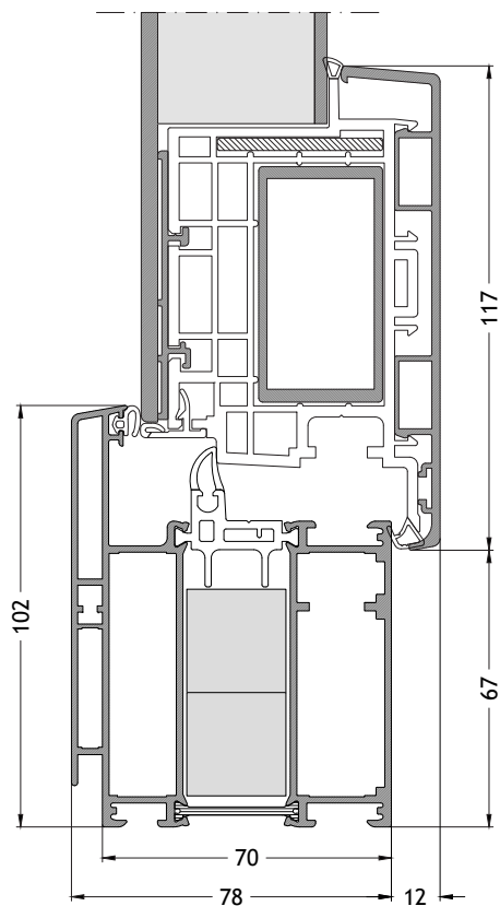
Telaio forma ad L 711 apertura verso l'interno con anta A95 Scala 1:2
