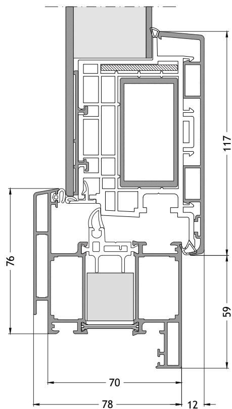
Telaio forma a Z/T 712 apertura verso l'interno con anta A95 Scala 1:2
