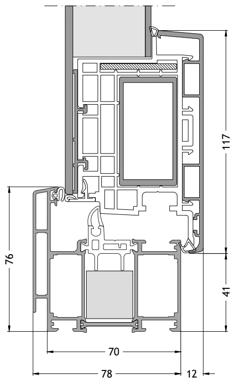
Telaio forma ad L 705 apertura verso l'interno con anta A95 Scala 1:2
