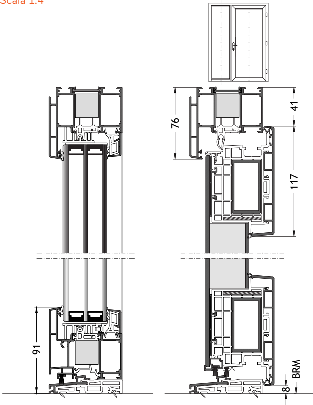
Soglia ribassata S0 apertura verso l'interno con anta A95 Scala 1:4
