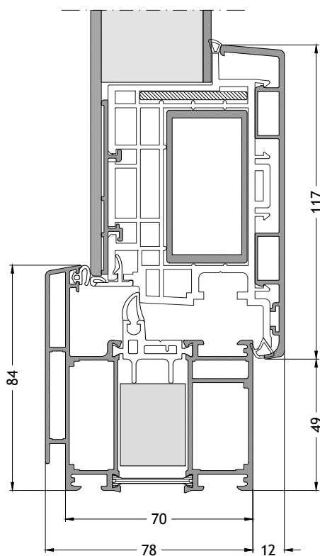
Telaio forma ad L 706 apertura verso l'interno con anta A95 Scala 1:2
