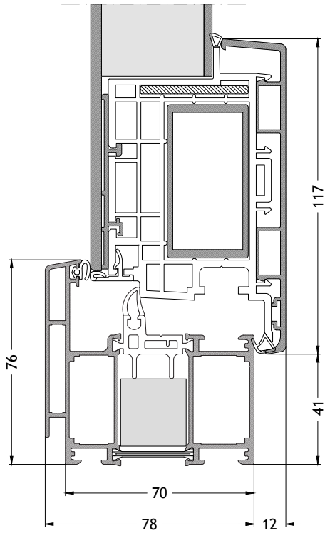
Blendrahmen L-Form 705 nach innen öffnend mit Flügel A95 Maßstab 1:2
