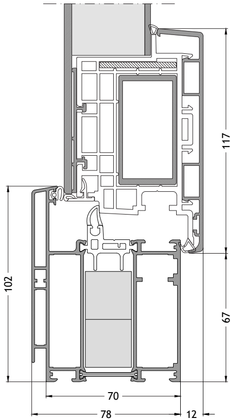
Blendrahmen L-Form 711 nach innen öffnend mit Flügel A95 Maßstab 1:2
