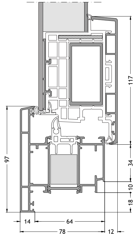
Blendrahmen Z-/T-Form 718 nach innen öffnend mit Flügel A95 Maßstab 1:2
