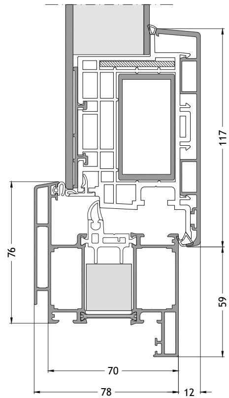
Blendrahmen Z-/T-Form 712 nach innen öffnend mit Flügel A95 Maßstab 1:2
