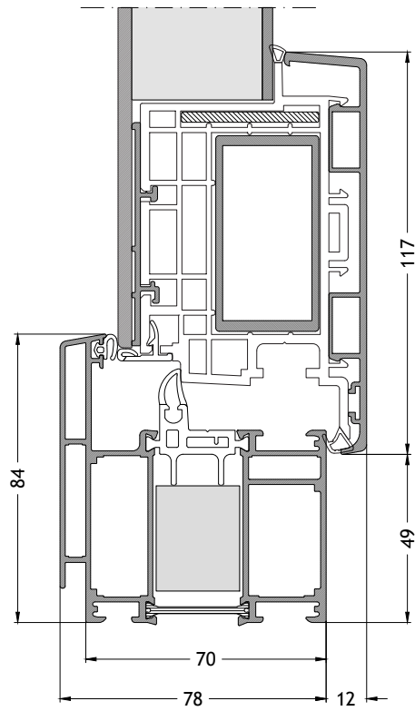
Blendrahmen L-Form 706 nach innen öffnend mit Flügel A95 Maßstab 1:2
