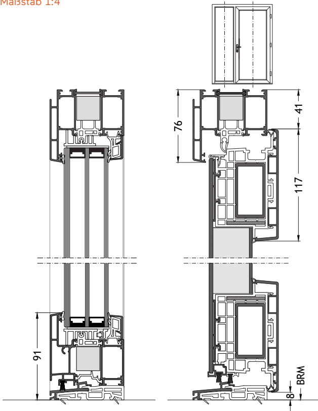
Flache Schwelle S0 nach innen öffnend mit Flügel A95 Maßstab 1:4
