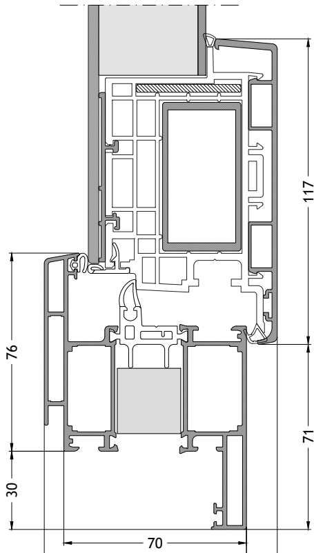
Blendrahmen Z-Form 719 nach innen öffnend mit Flügel A95 Maßstab 1:2
