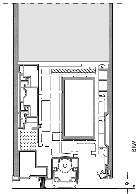
Seuil plat S4 ouverture vers l'intérieur avec ouvrant F96 Échelle 1:2
