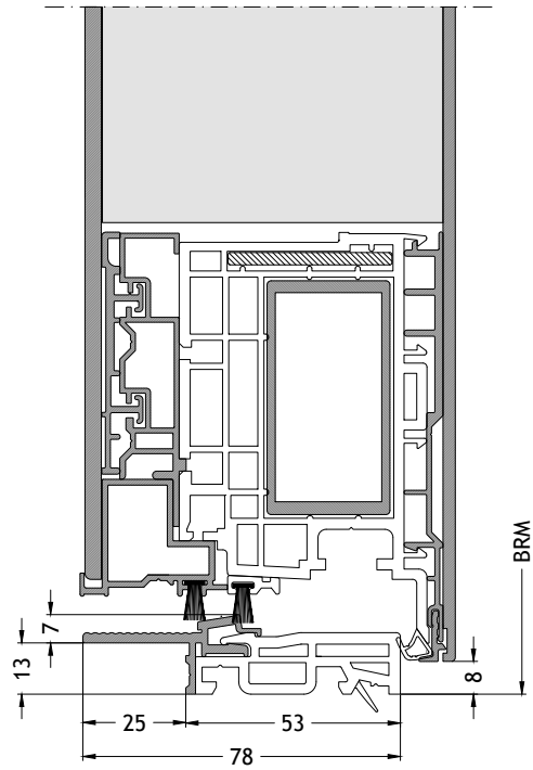
Seuil plat S2 ouverture vers l'intérieur avec ouvrant F96 Échelle 1:2
