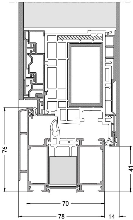
Dormant en L 705 ouverture vers l'intérieur avec ouvrant F96 Échelle 1:2
