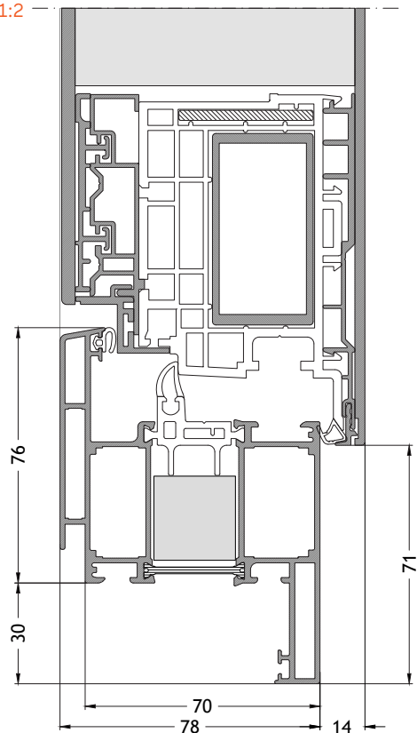
Dormant en Z 719 ouverture vers l'intérieur avec ouvrant F96 Échelle 1:2
