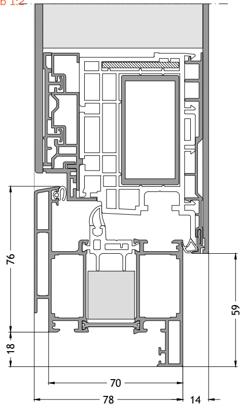
Dormant en Z/T 712 ouverture vers l'intérieur avec ouvrant F96 Maßstab 1:2
