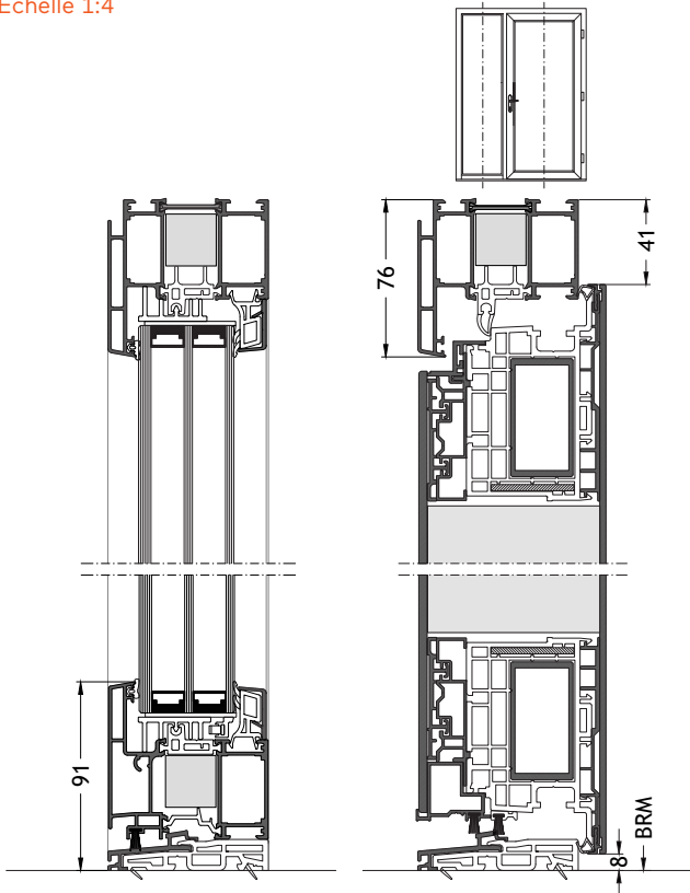
Seuil plat S0 ouverture vers l'intérieur avec ouvrant F96 Échelle 1:4
