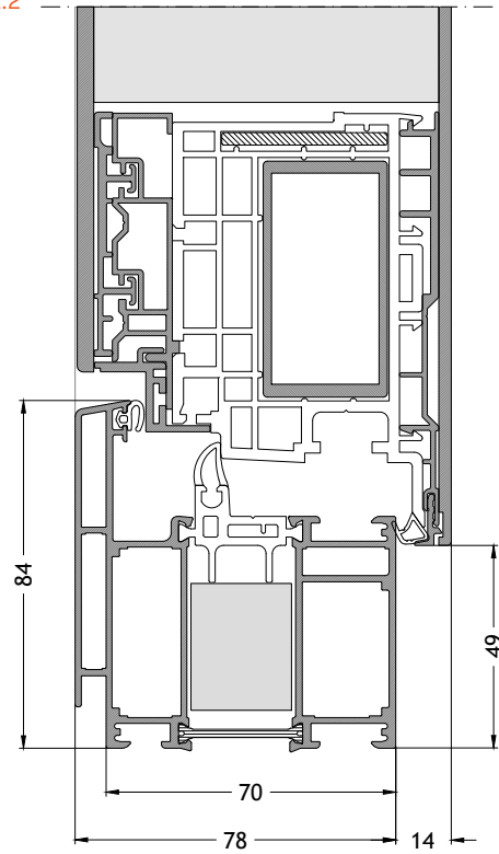
Dormant en L 706 ouverture vers l'intérieur avec ouvrant F96 Échelle 1:2
