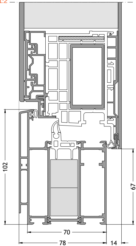
Dormant en L 711 ouverture vers l'intérieur avec ouvrant F96 Échelle 1:2
