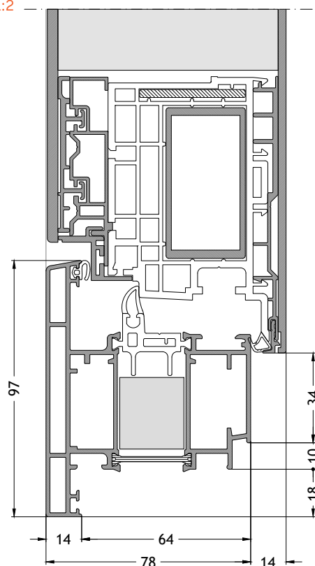
Dormant en Z/T 718 ouverture vers l'intérieur avec ouvrant F96 Échelle 1:2
