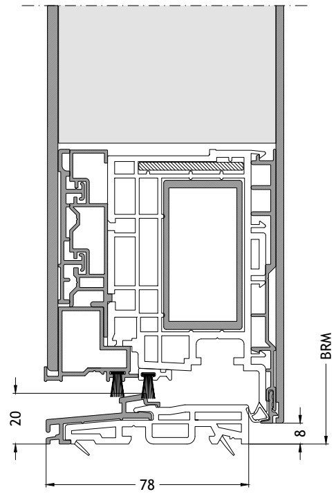
Seuil plat S0 ouverture vers l'intérieur avec ouvrant F96 Échelle 1:2
