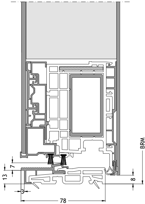
Seuil plat S1 ouverture vers l'intérieur avec ouvrant F96 Échelle 1:2
