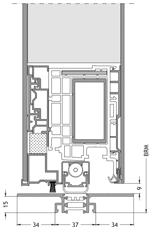
Seuil plat S3 ouverture vers l'intérieur avec ouvrant F96 Échelle 1:2
