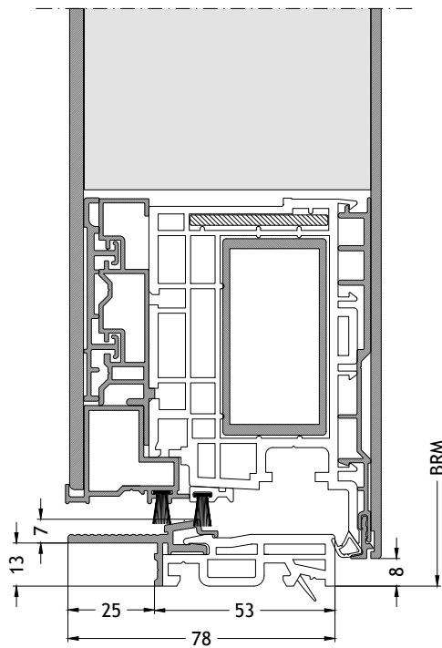
Soglia ribassata S2 apertura verso l'interno con anta F96
