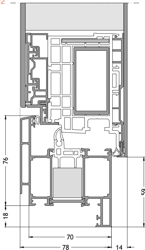
Telaio forma a Z/T 712 apertura verso l'interno con anta F96 Scala 1:2
