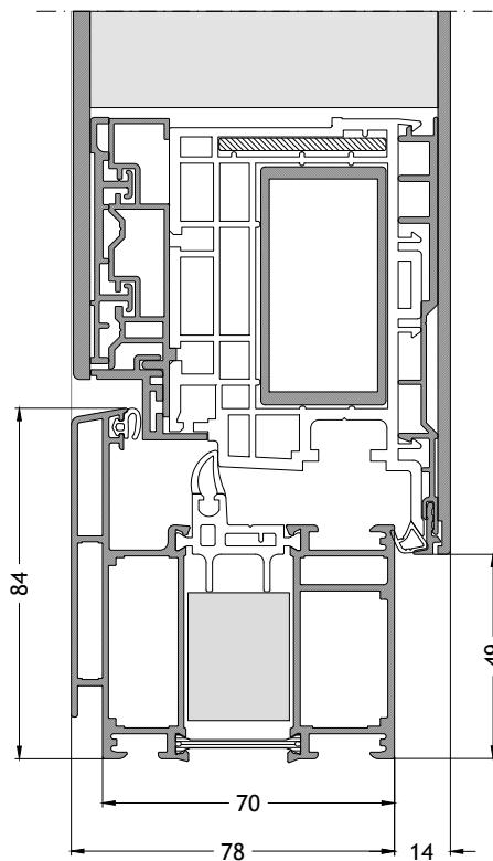
Telaio forma ad L 706 apertura verso l'interno con anta F96 Scala 1:2
