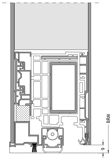
Soglia ribassata S4 apertura verso l'interno con anta F96 Scala 1:2
