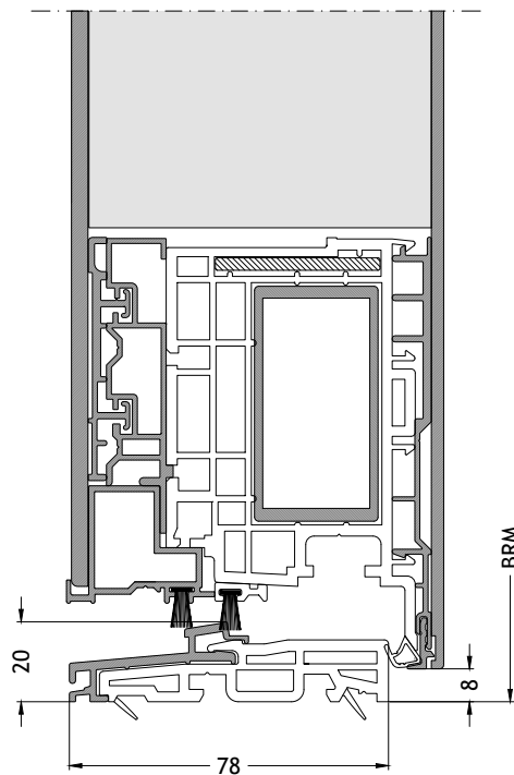
Soglia ribassata S0 apertura verso l'interno con anta F96
