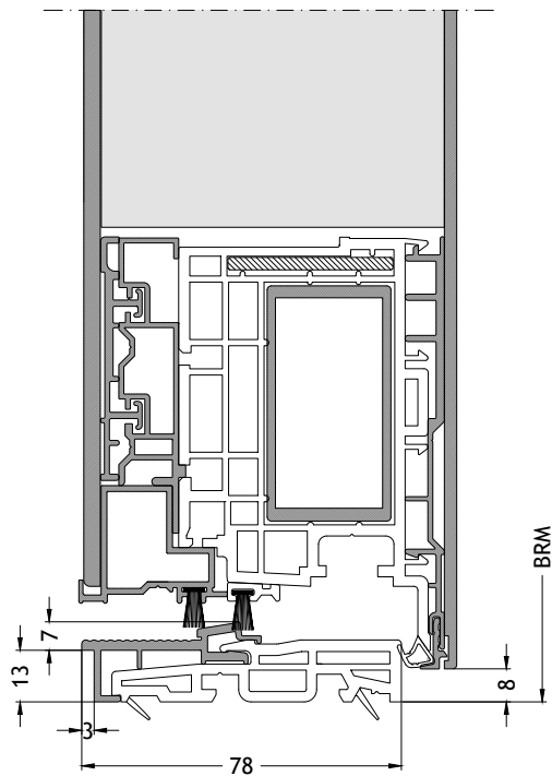
Soglia ribassata S1 apertura verso l'interno con anta F96
