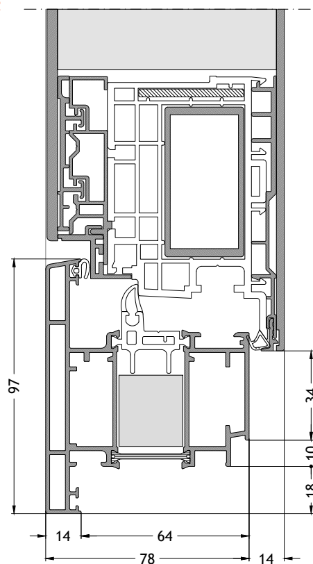
Telaio forma a Z/T 718 apertura verso l'interno con anta F96 Scala 1:2
