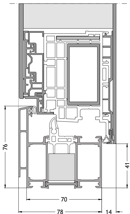
Telaio forma ad L 705 apertura verso l'interno con anta F96 Scala 1:2
