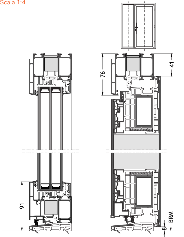
Soglia ribassata S0 apertura verso l'interno con anta F96
