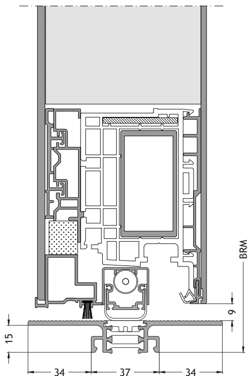
Soglia ribassata S3 apertura verso l'interno con anta F96 Scala 1:2
