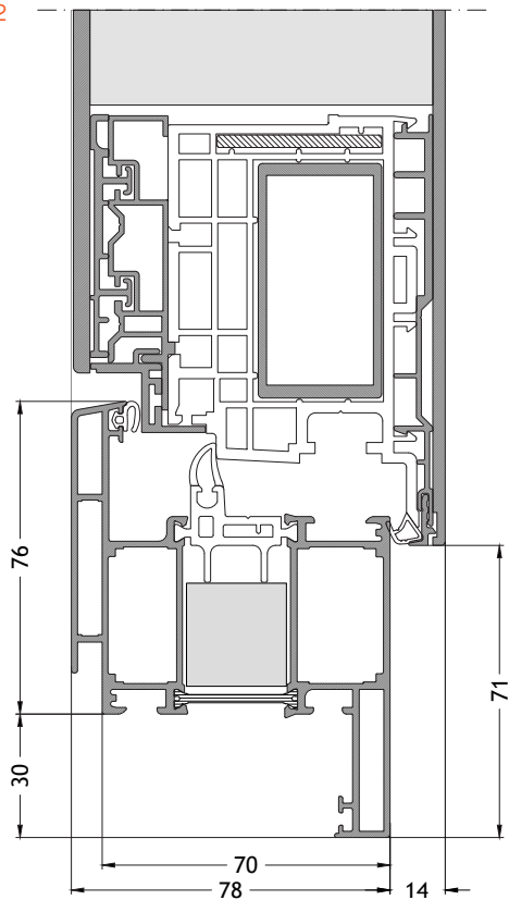
Telaio forma a Z 719 apertura verso l'interno con anta F96 Scala 1:2
