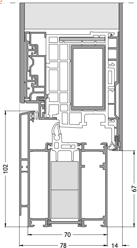
Telaio forma ad L 711 apertura verso l'interno con anta F96 Scala 1:2
