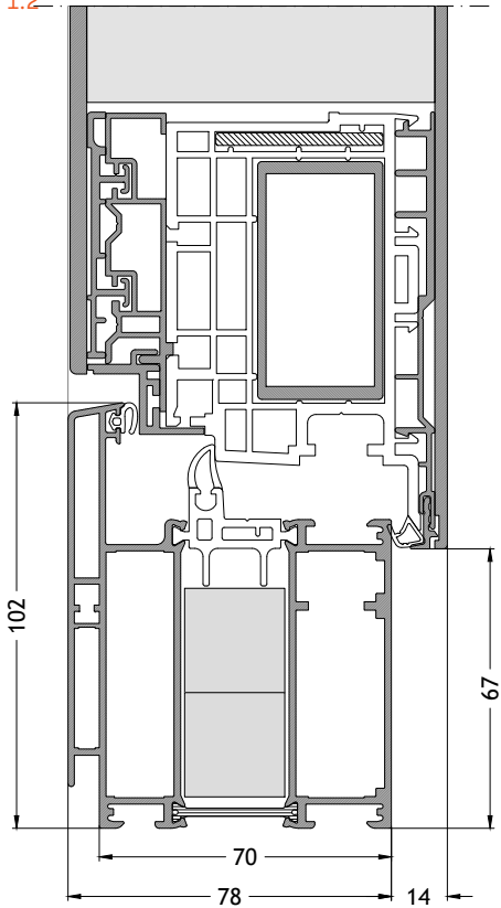
Blendrahmen L-Form 711 nach innen öffnend mit Flügel F96 Maßstab 1:2
