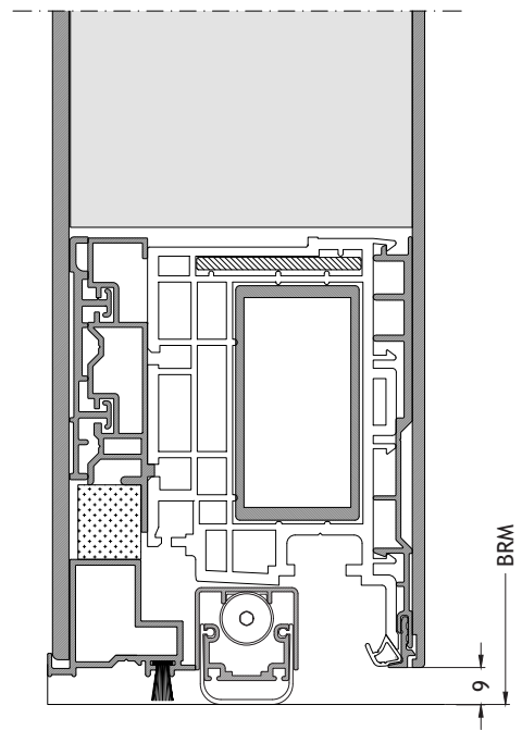
Flache Schwelle S4 nach innen öffnend mit Flügel F96 Maßstab 1:2
