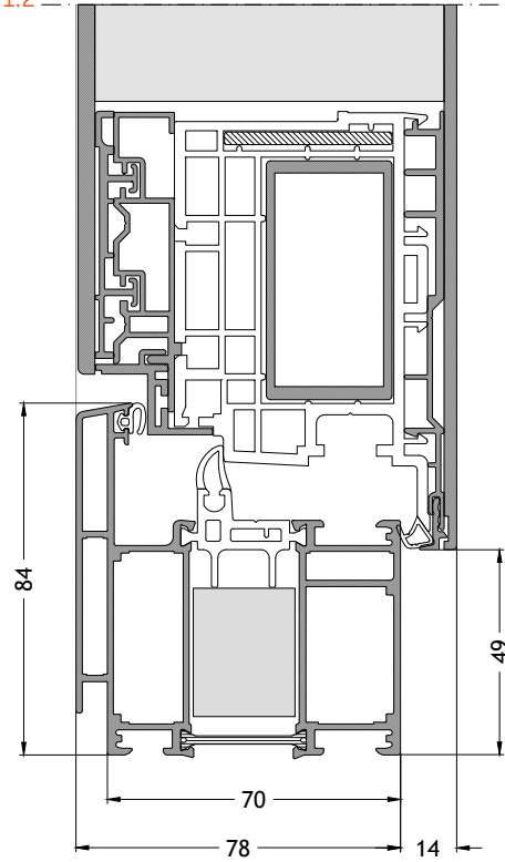
Blendrahmen L-Form 706 nach innen öffnend mit Flügel F96 Maßstab 1:2
