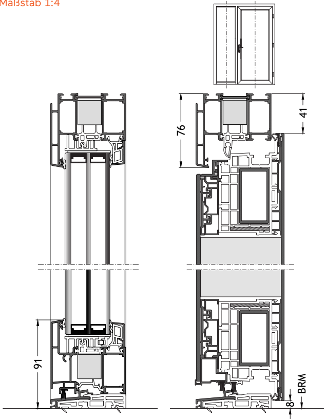
Flache Schwelle S0 nach innen öffnend mit Flügel F96 Maßstab 1:4
