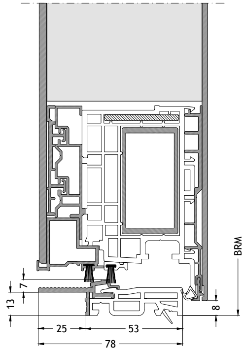
Flache Schwelle S2 nach innen öffnend mit Flügel F96 Maßstab 1:2
