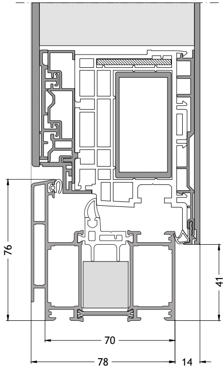
Blendrahmen L-Form 705 nach innen öffnend mit Flügel F96 Maßstab 1:2
