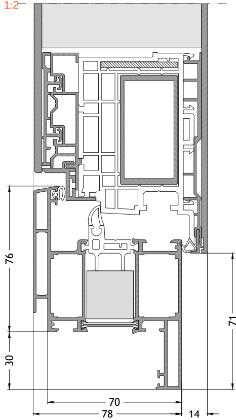
Blendrahmen Z-Form 719 nach innen öffnend mit Flügel F96 Maßstab 1:2
