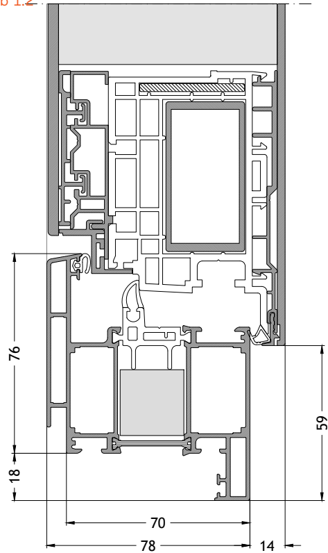
Blendrahmen Z-/T-Form 712 nach innen öffnend mit Flügel F96 Maßstab 1:2
