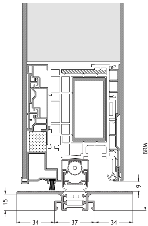
Flache Schwelle S3 nach innen öffnend mit Flügel F96 Maßstab 1:2
