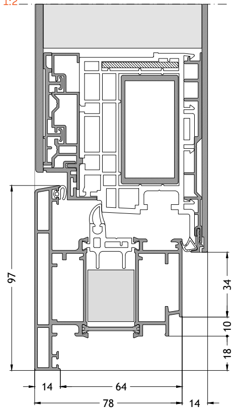
Blendrahmen Z-/T-Form 718 nach innen öffnend mit Flügel F96 Maßstab 1:2
