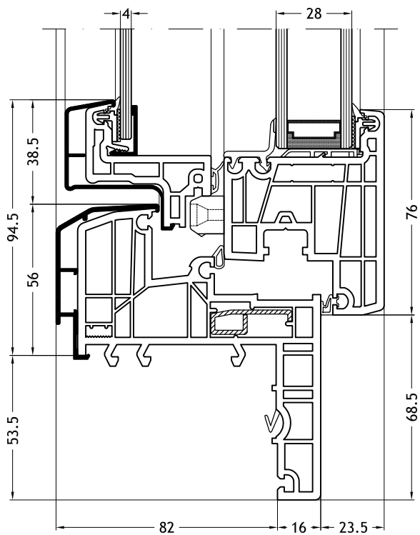
Telaio a Z 929K con anta Slim-line Twin C
