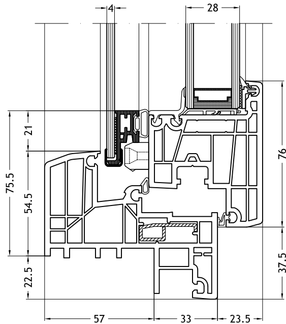
Telaio a Z 921 con anta Nova-line Twin
