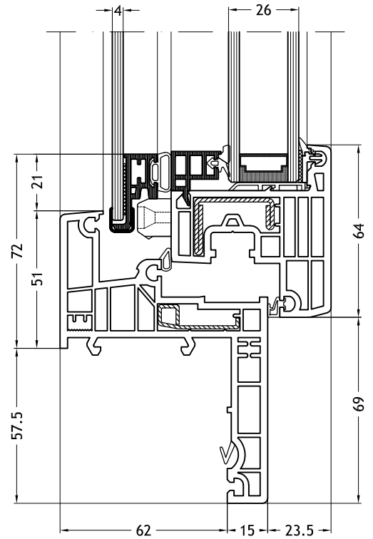
Kozijn Z-vorm 966 met vleugel Nova-line Twin
