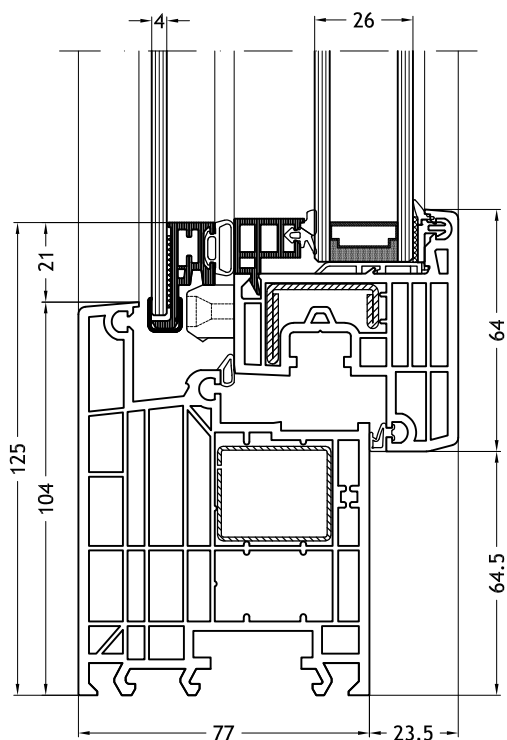
Kozijn L-vorm 963 met vleugel Nova-line Twin
