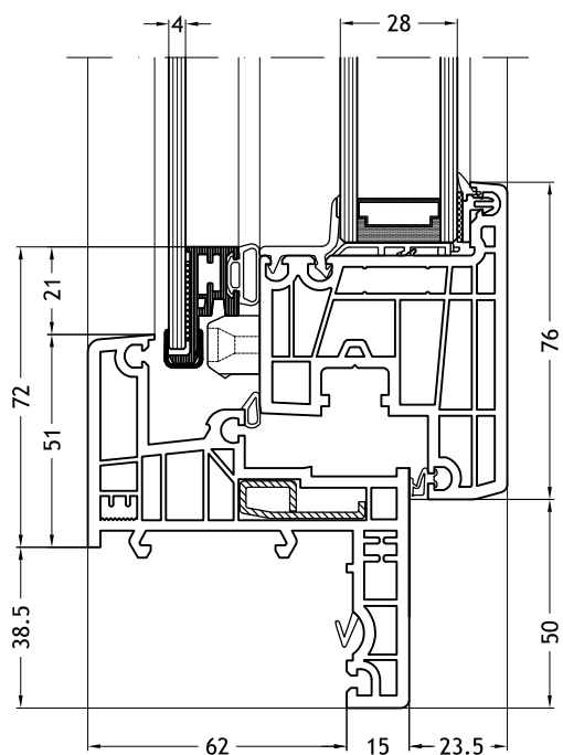
Dormant en Z, 965 avec ouvrant Nova-line Twin
