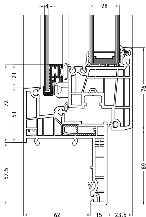
Telaio a Z 966 con anta Nova-line Twin
