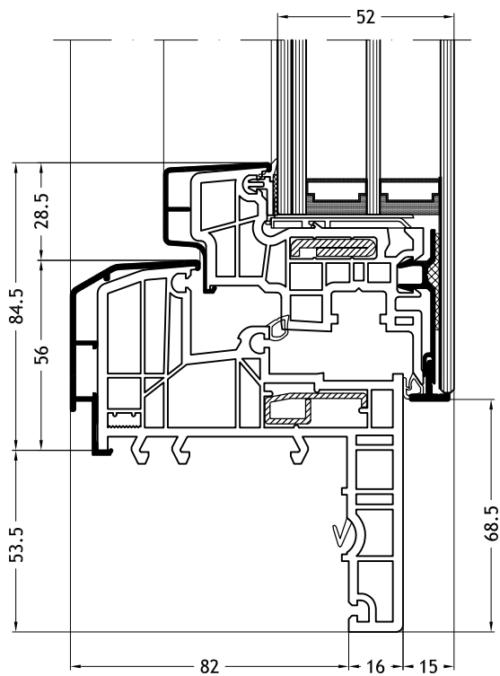
Marco Z - 929K con hoja Slim-line Cristal C
