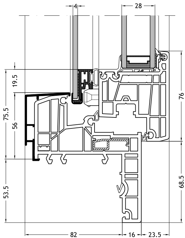
Telaio monoblocco a Z 929N con anta Nova-line Twin N
