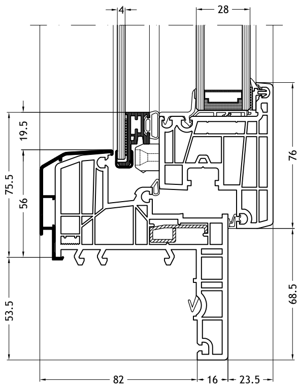
Dormant en Z, 929K avec ouvrant Nova-line Twin C
