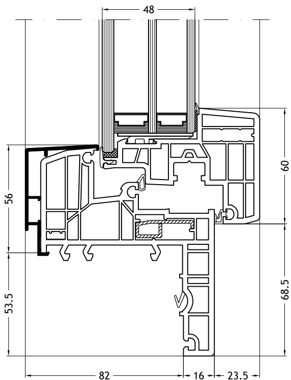
Dormant en Z, 929N avec ouvrant Nova-line Plus N
