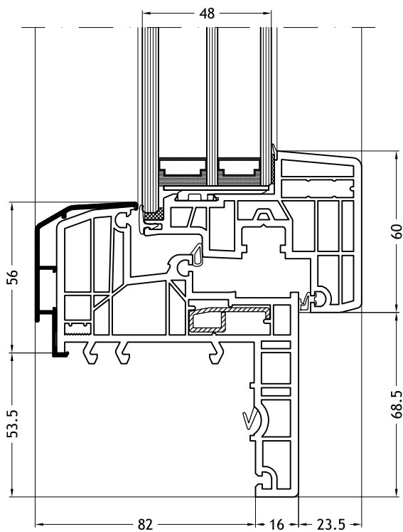
Dormant en Z, 929K avec ouvrant Nova-line Plus C
