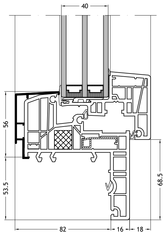
Vlakte onderdorpel met vleugel Nova-line C 953
