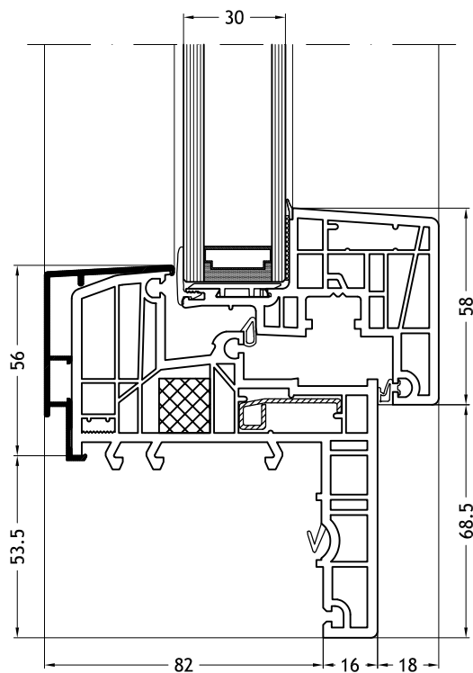
Vlakte onderdorpel met vleugel Nova-line C 971
