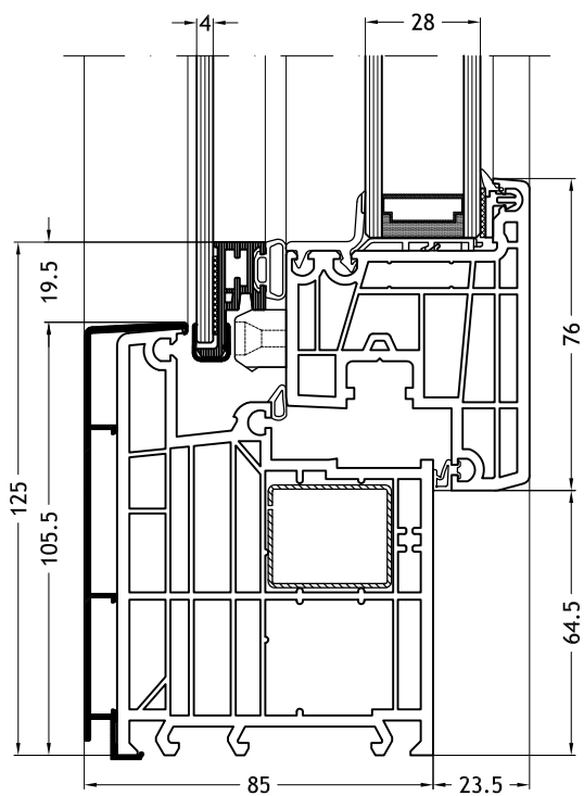
Marco L - 963N con hoja Nova-line Twin
