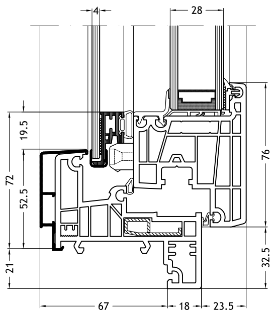
Marco Z, 964N con hoja Nova-line Twin
