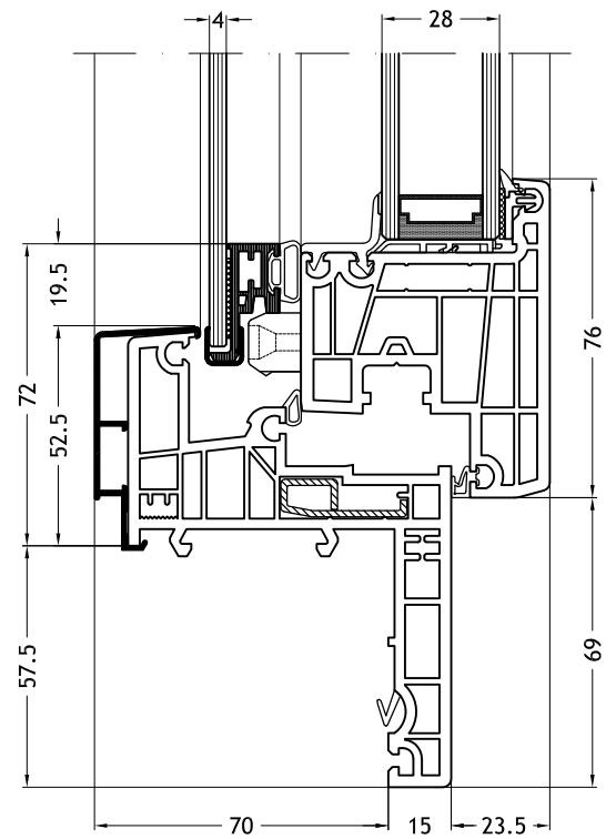
Dormant en Z, 966N avec ouvrant Nova-line Twin
