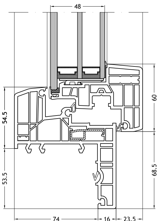
Marco Z, 929 con hoja Nova-line Plus
