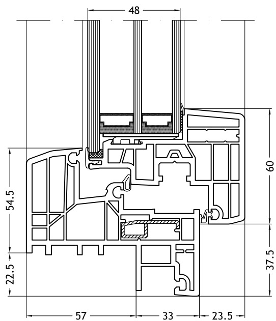
Marco Z, 921 con hoja Nova-line Plus
