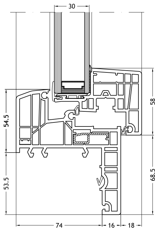
Seuil plat avec ouvrant Nova-line 971
