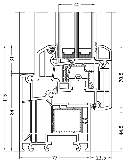
Marco L - 962 con hoja Step-line
