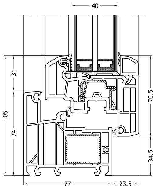
Marco L - 961 con hoja Step-line
