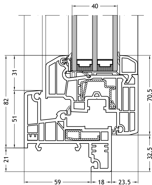
Marco Z, 964 con hoja Step-line
