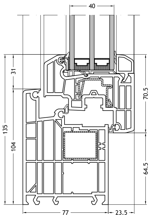
Marco L, 963 con hoja Step-line
