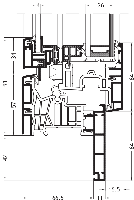
Kozijn Z-vorm D2V met vleuge Slim-line Twin A31
