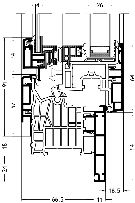
Kozijn L-vorm D1Y met vleuge Slim-line Twin A31
