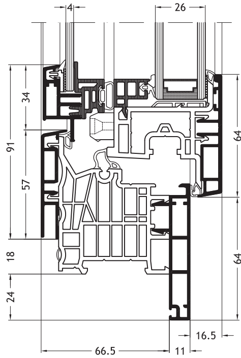
Kozijn L-vorm D1V met vleuge Slim-line Twin A31
