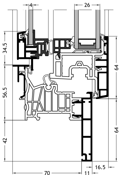
Kozijn Z-vorm D2X met vleuge Slim-line Twin A31
