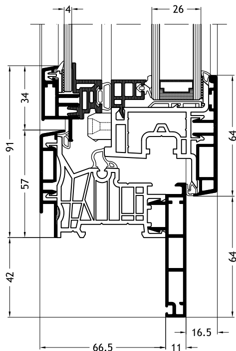
Kozijn Z-vorm D2Y met vleuge Slim-line Twin A31
