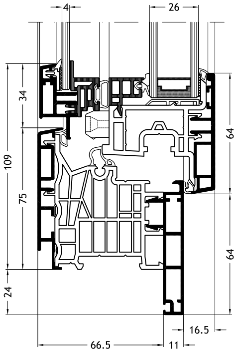
Kozijn L-vorm D1Z met vleuge Slim-line Twin A31
