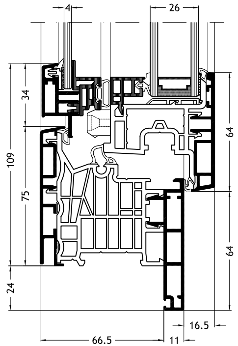
Kozijn L-vorm D1W met vleuge Slim-line Twin A31
