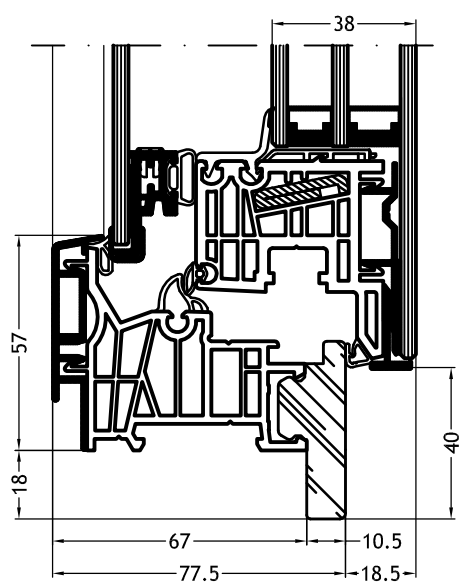
Kozijn Z-vorm 9A2Y met vleugel Nova-line Cristal Twin
