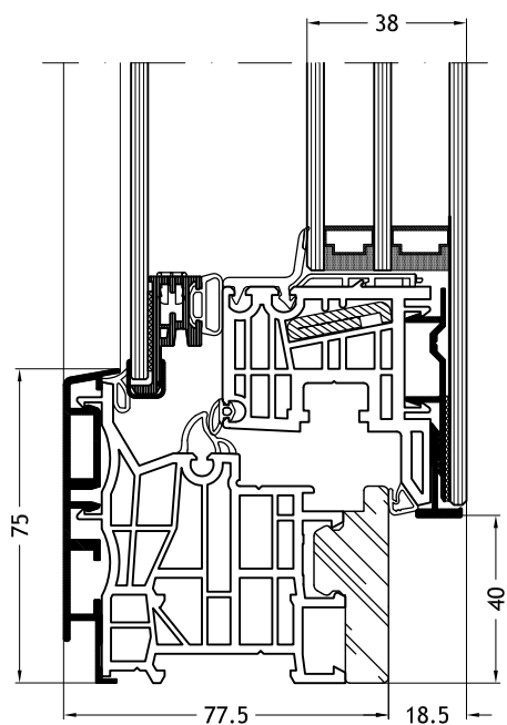
Kozijn L-vorm 9A1Z met vleugel Nova-line Cristal Twin
