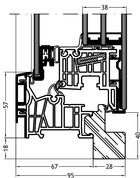
Kozijn Z-vorm 9F2Y met vleugel Nova-line Cristal Twin
