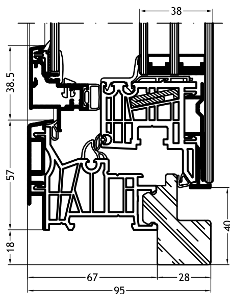
Kozijn Z-vorm 9F2Y met vleugel Classic-line Cristal Twin
