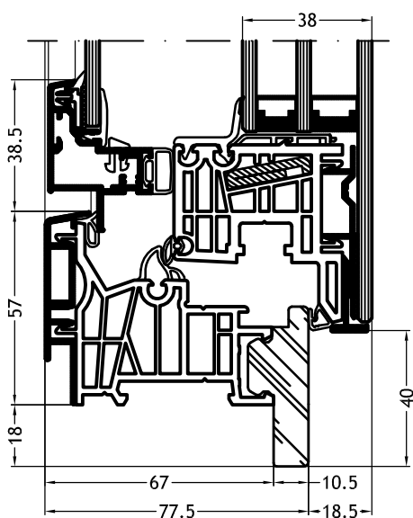
Kozijn Z-vorm 9A2Y met vleugel Classic-line Cristal Twin
