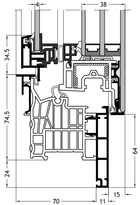
Blendrahmen L-Form D1X mit Flügel Slim-line Cristal Twin A33
