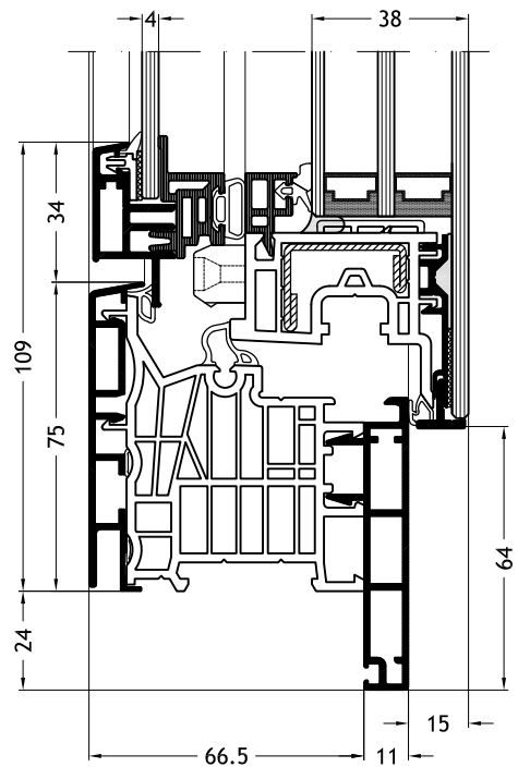
Blendrahmen L-Form D1W mit Flügel Slim-line Cristal Twin A33
