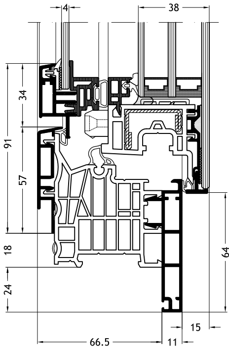
Blendrahmen L-Form D1Y mit Flügel Slim-line Cristal Twin A33
