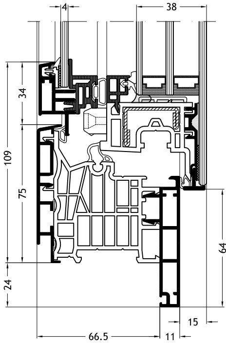
Blendrahmen L-Form D1Z mit Flügel Slim-line Cristal Twin A33
