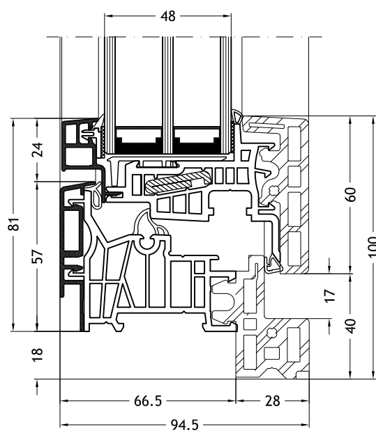
Dormant en Z, 8F2Y avec ouvrant Classic-line
