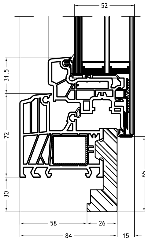
Marco Z - 9D60 con hoja Slim-line Cristal
