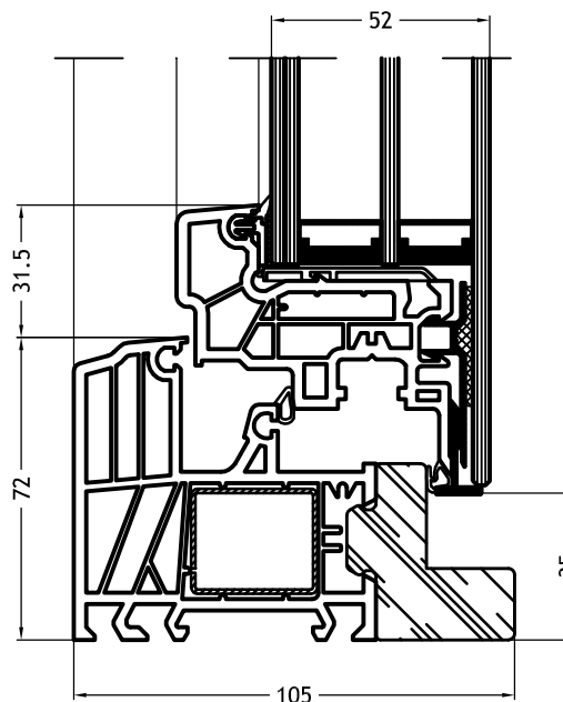
Marco L - 9F60 con hoja Slim-line Cristal
