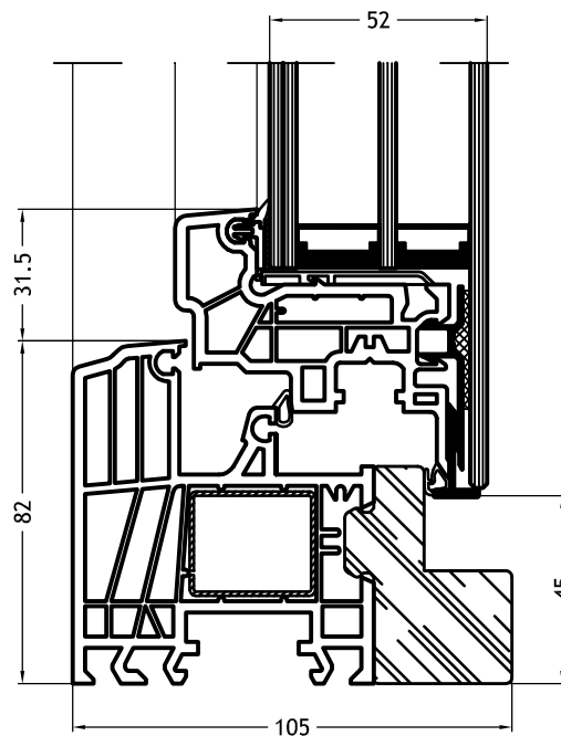
Marco L - 9G43 con hoja Slim-line Cristal
