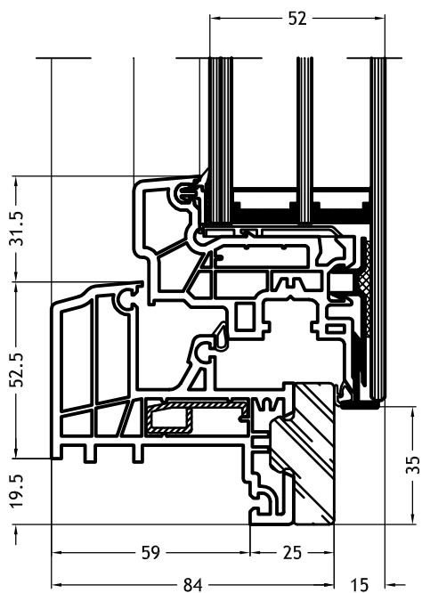
Marco Z - 9A36 con hoja Slim-line Cristal
