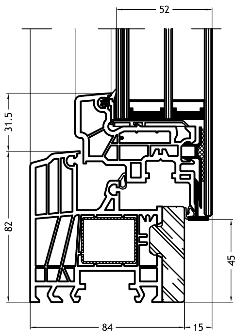
Marco L - 9B43 con hoja Slim-line Cristal
