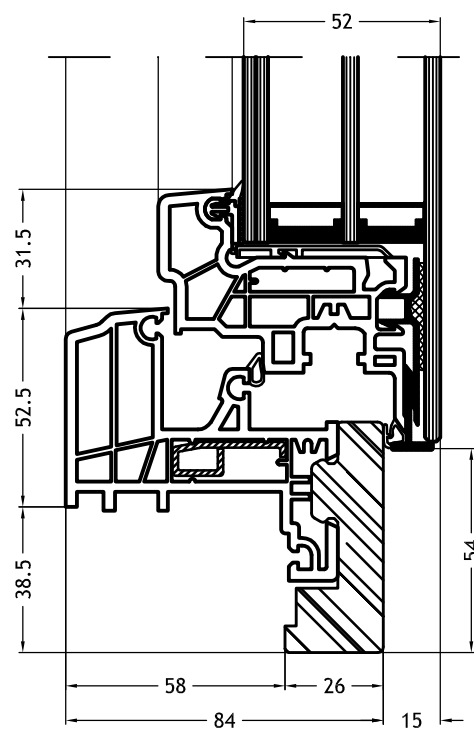
Marco Z - 9E36 con hoja Slim-line Cristal
