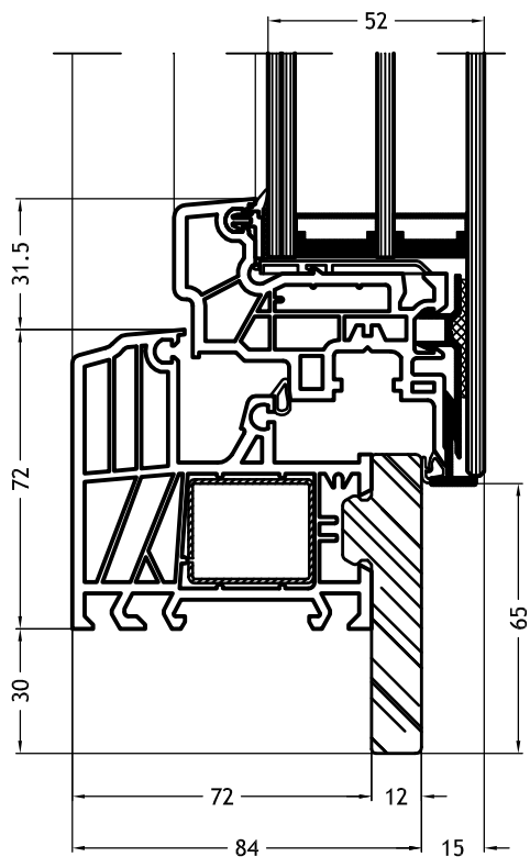
Marco Z - 9C60 con hoja Slim-line Cristal
