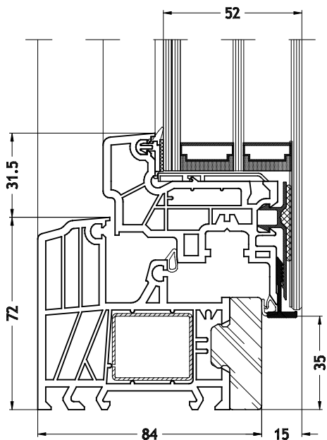
Marco L - 9A60 con hoja Slim-line Cristal
