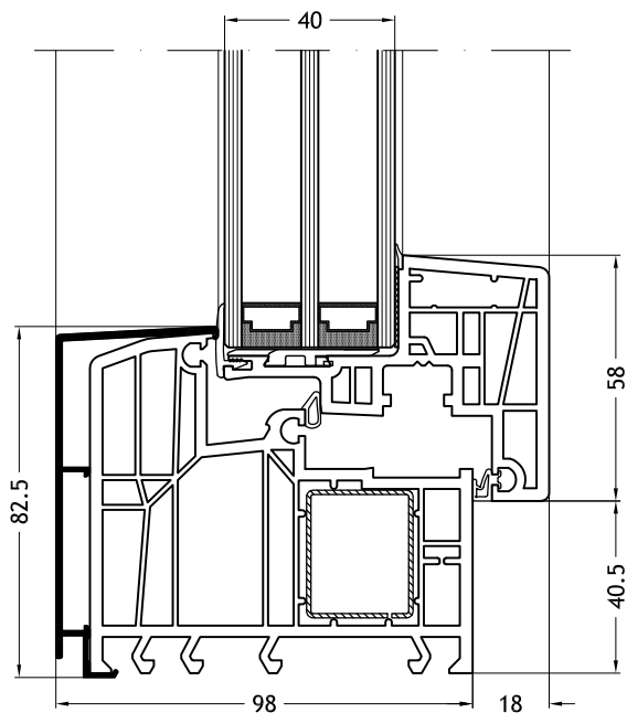
Marco L - 920N con hoja Nova-line N
