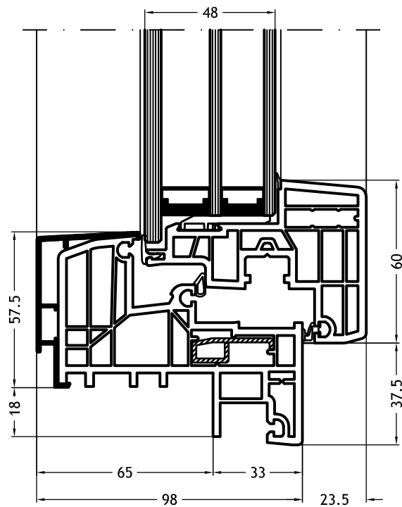
Marco Z - 921N con hoja Nova-line N
