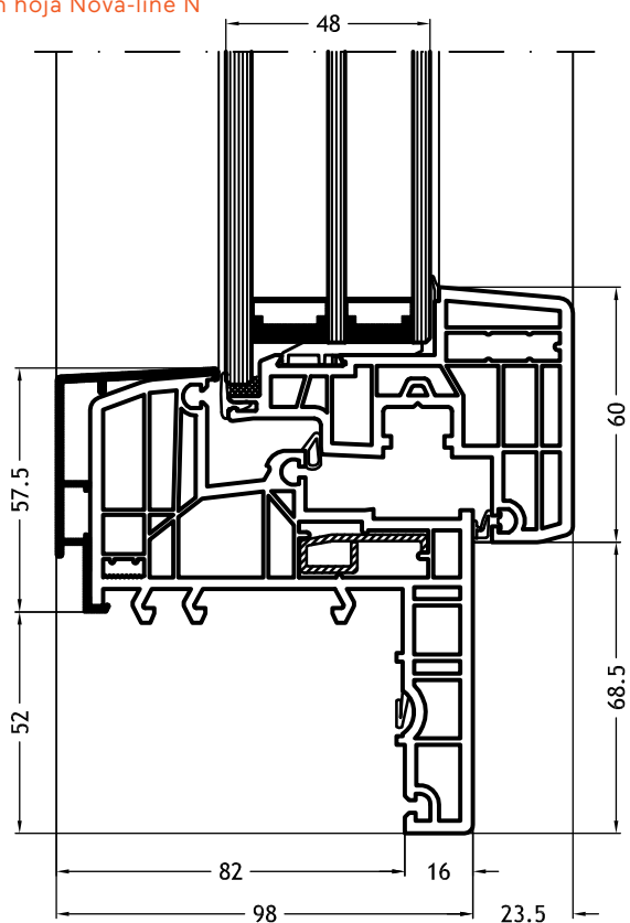
Marco Z - 929N con hoja Nova-line N
