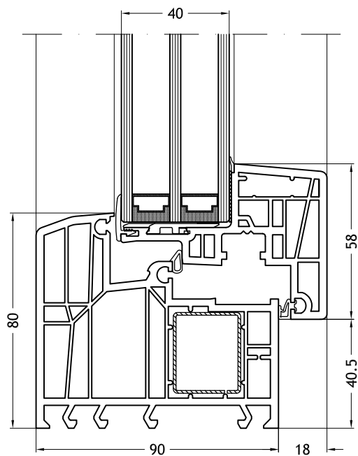
Kozijn L-vorm 920 met vleugel Nova-line
