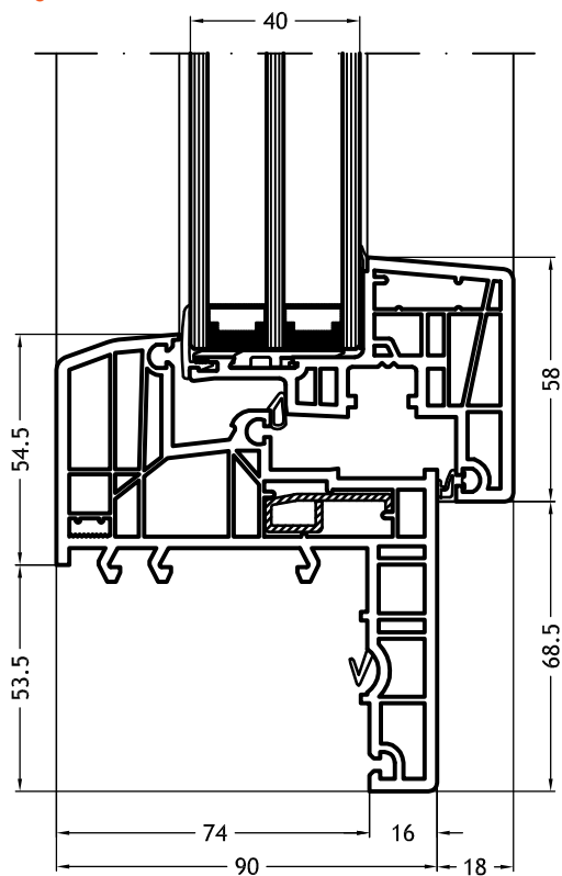
Kozijn Z-vorm 929 met vleugel Nova-line
