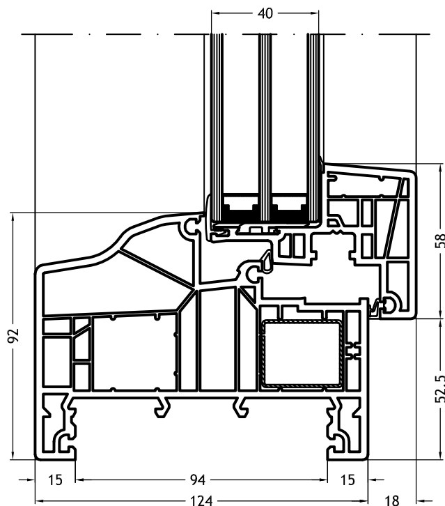
Blok-kozijn L-vorm 951 met vleugel Nova-line
