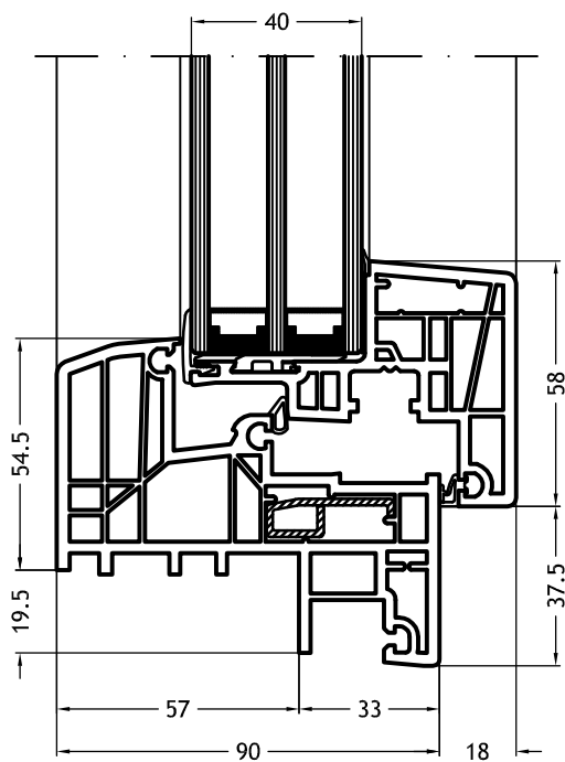
Kozijn Z-vorm 921 met vleugel Nova-line
