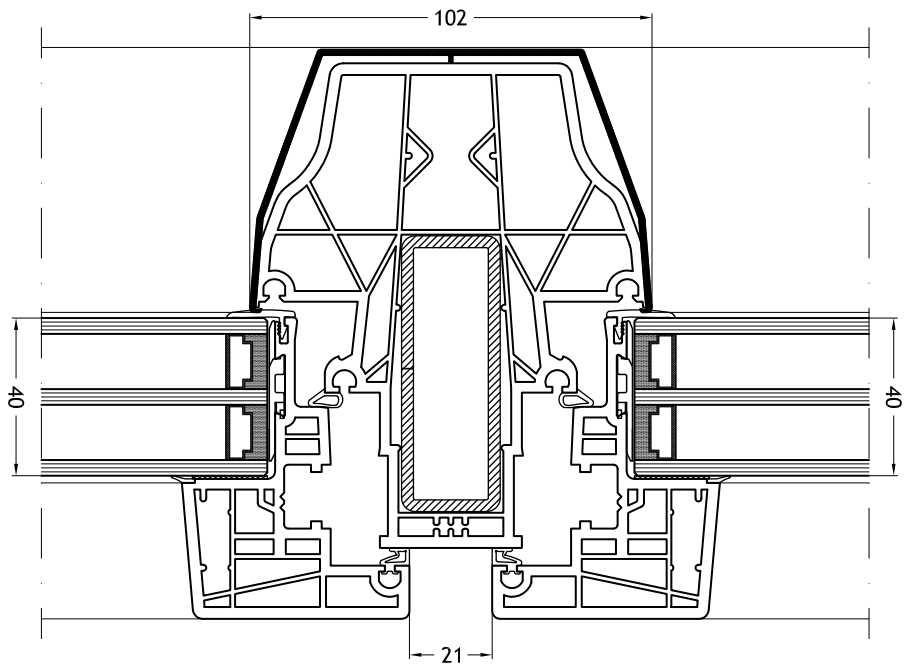
Kalf/Stijl 952K voor blok-kozijn met vleugel Nova-line C
