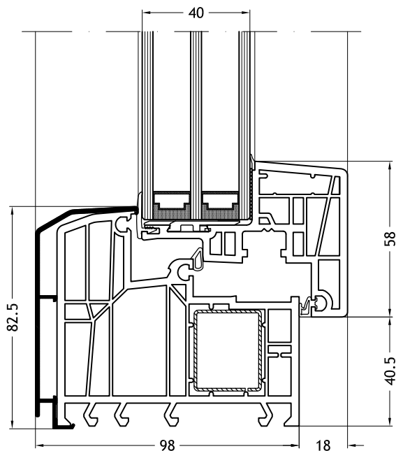
Kozijn L-vorm 920K met vleugel Nova-line C
