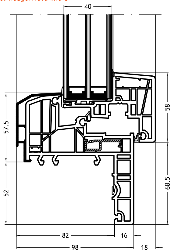
Kozijn Z-vorm 929K met vleugel Nova-line C
