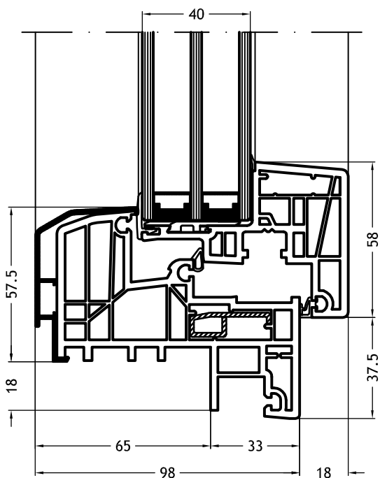
Kozijn Z-vorm 921K met vleugel Nova-line C
