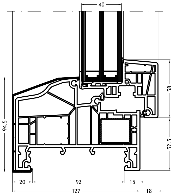
Blok-kozijn L-vorm 951K met vleugel Nova-line C
