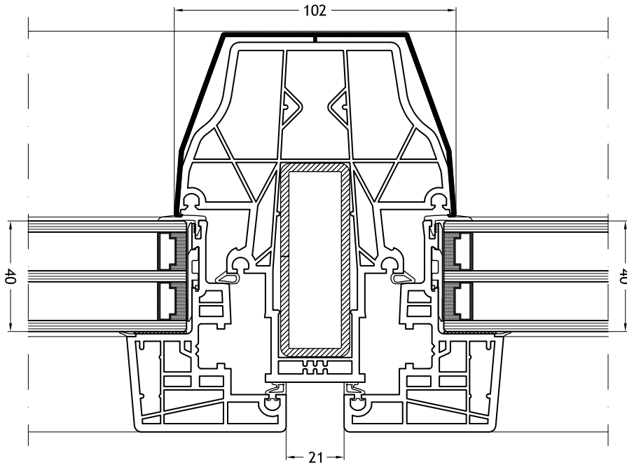
Travesaño 952 para marco bloc con hoja Nova-line C
