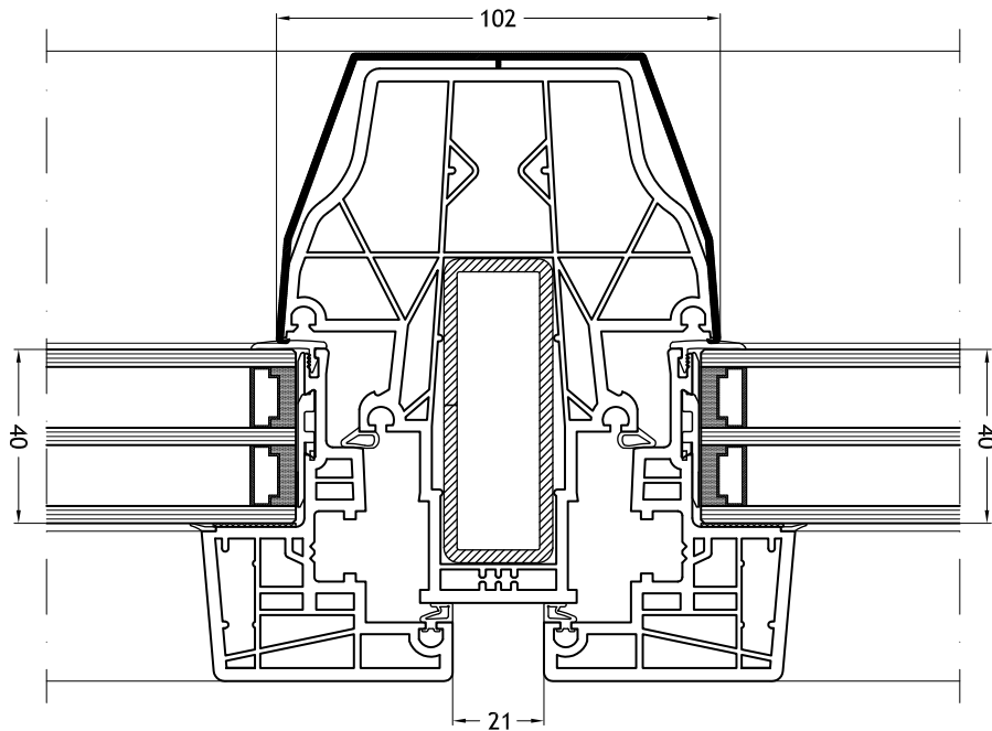
Montant/traverse 952K pour dormant bloc avec ouvrant Nova-line C
