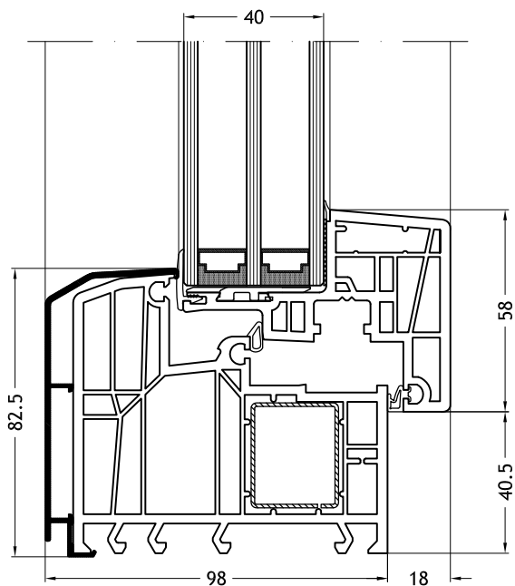
Dormant en L, 920K avec ouvrant Nova-line C
