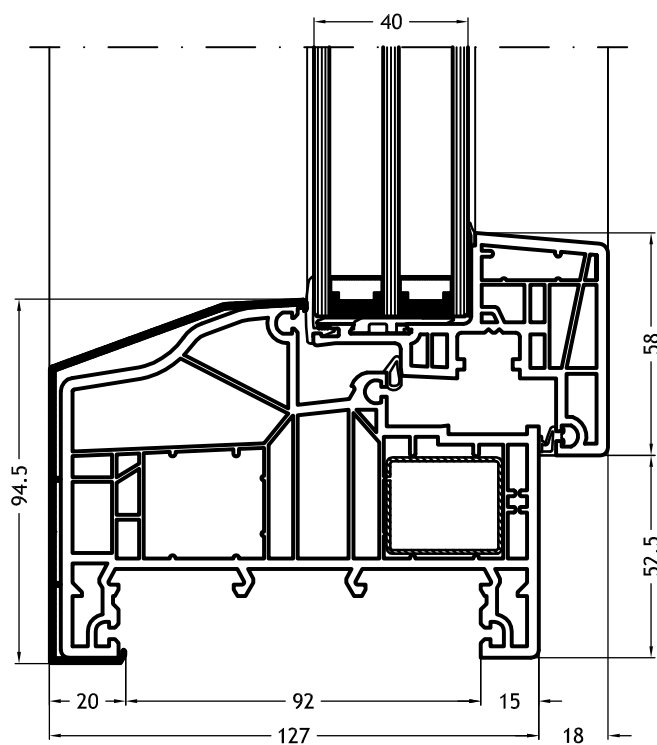
Dormant bloc en L, 951K avec ouvrant Nova-line C
