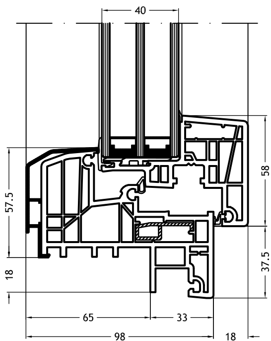
Dormant en Z, 921K avec ouvrant Nova-line C
