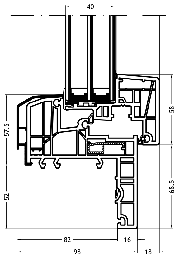
Dormant en Z, 929K avec ouvrant Nova-line C
