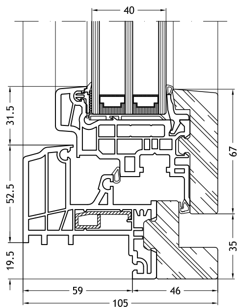
Kozijn Z-vorm 9F36 met vleugel Slim-line 9086
