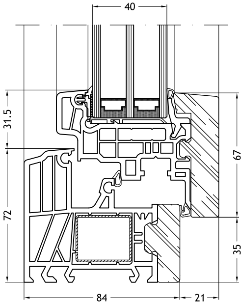
Kozijn L-vorm 9A60 met vleugel Slim-line 9086
