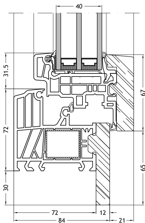
Kozijn Z-vorm 9C60 met vleugel Slim-line 9086
