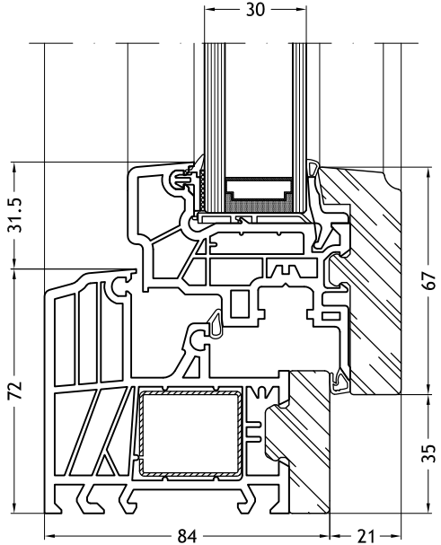
Kozijn L-vorm 9A60 met vleugel Slim-line 9S87 met glaslat stijl
