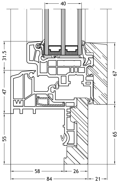
Kozijn Z-vorm 9D63 met vleugel Slim-line 9086
