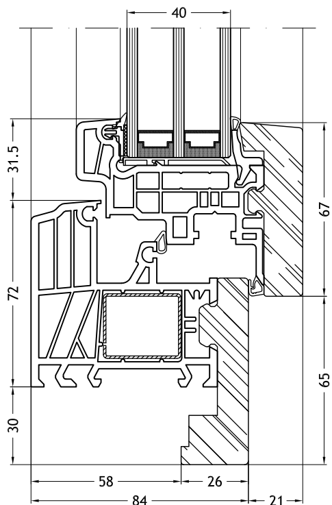
Kozijn Z-vorm 9D60 met vleugel Slim-line 9086
