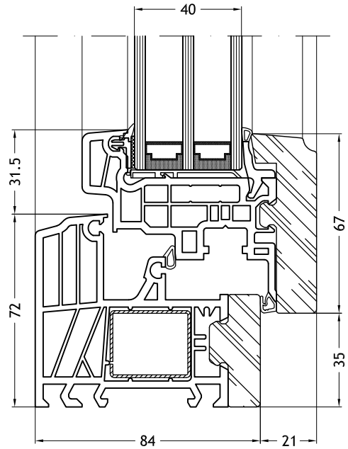
Kozijn L-vorm 9A60 met vleugel Slim-line 9S86 met glaslat stijl
