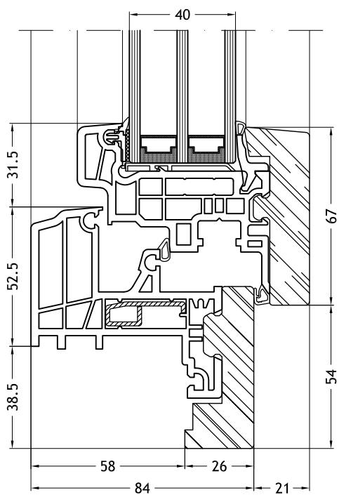
Kozijn Z-vorm 9E36 met vleugel Slim-line 9086
