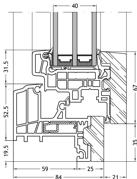
Kozijn Z-vorm 9A36 met vleugel Slim-line 9086
