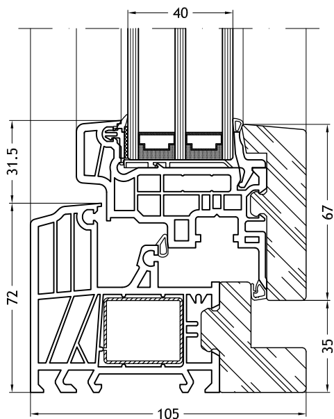
Kozijn L-vorm 9F60 met vleugel Slim-line 9086
