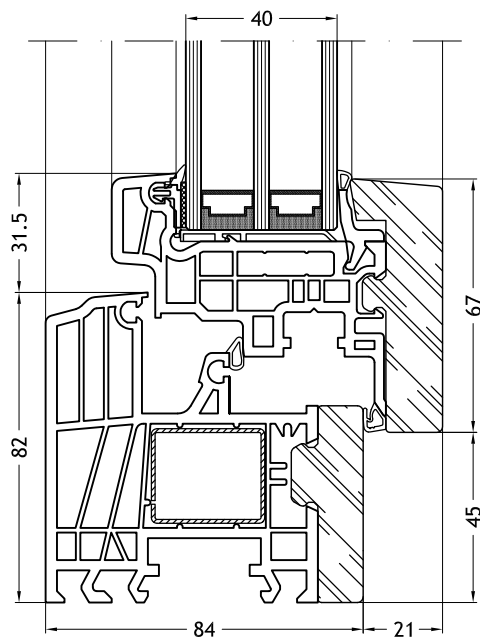
Kozijn L-vorm 9B43 met vleugel Slim-line 9086
