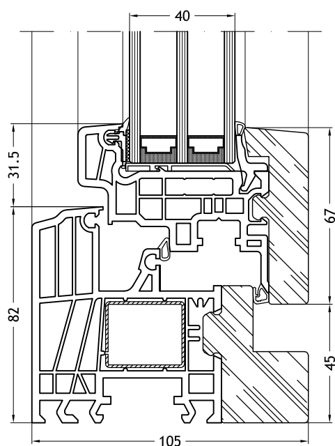
Kozijn L-vorm 9G43 met vleugel Slim-line 9086
