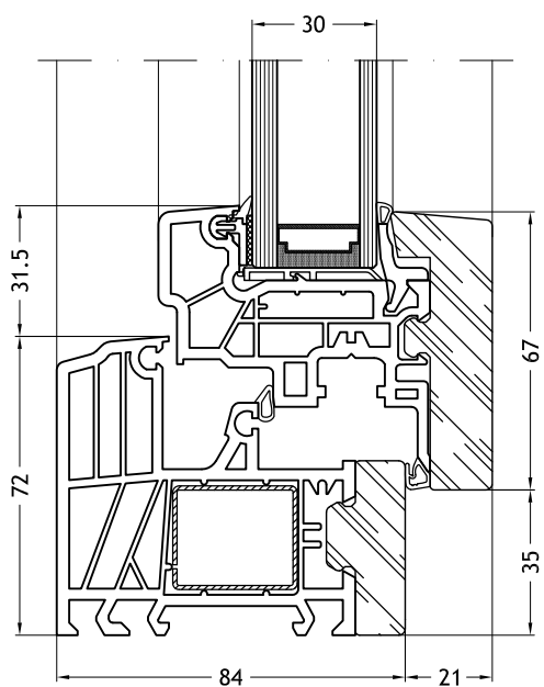
Marco L - 9A60 con hoja Slim-line 9087
