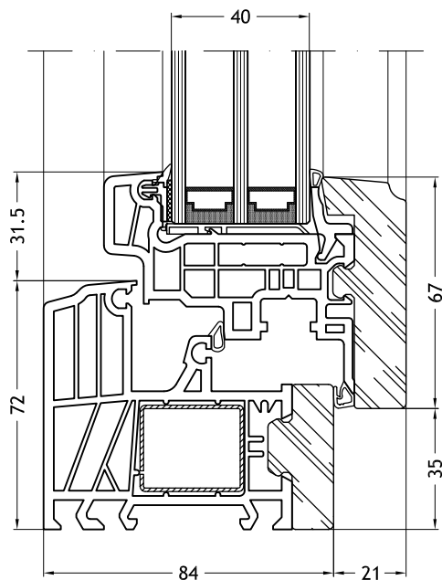
Marco L - 9A60 con hoja Slim-line 9S86 con acabado en Stilo
