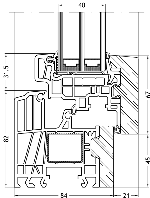
Marco L - 9B43 con hoja Slim-line 9086
