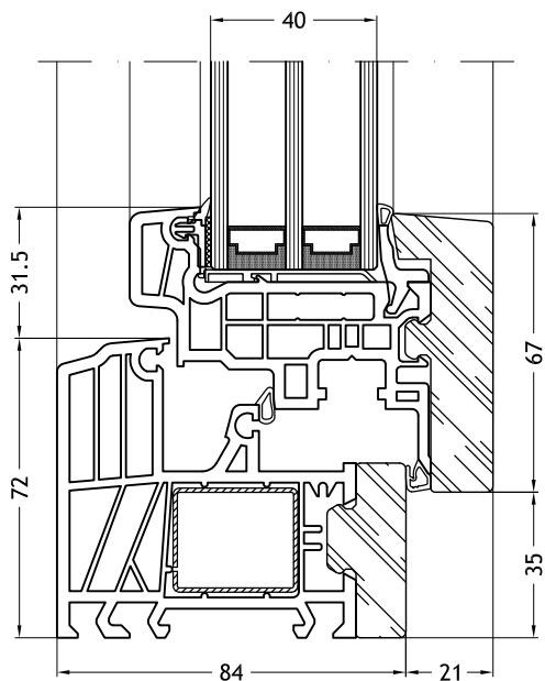
Marco L - 9A60 con hoja Slim-line 9086
