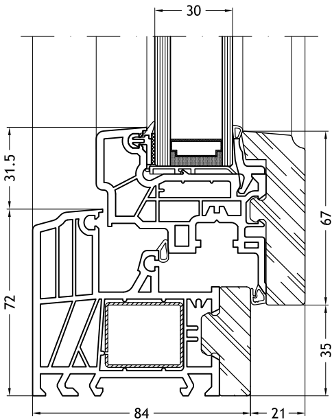
Marco L - 9A60 con hoja Slim-line 9S87 con acabado en Stilo
