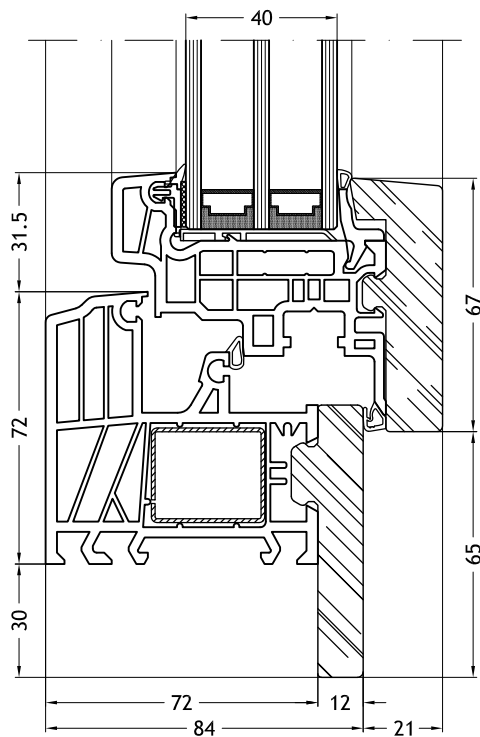
Marco Z - 9C60 con hoja Slim-line 9086
