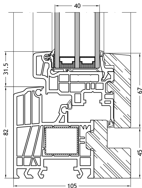
Marco L - 9G43 con hoja Slim-line 9086
