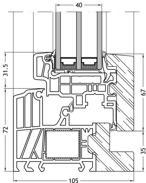
Marco L - 9F60 con hoja Slim-line 9086
