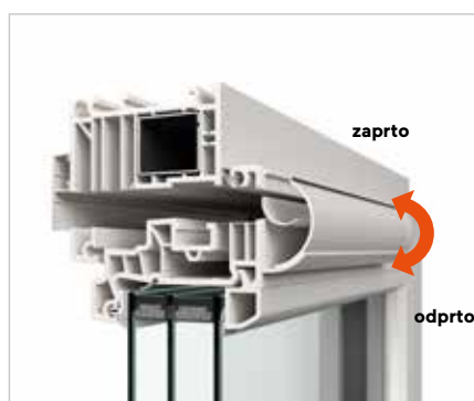
Okenski prezračevalnik PassiveVent Midi s sistemom za nadzor vlage ali brez njega
