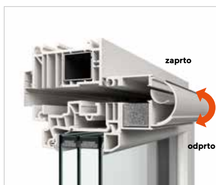
Okenski prezračevalnik PassiveVent Midi s sistemom za nadzor vlage in modulom za zvočno izolacijo
