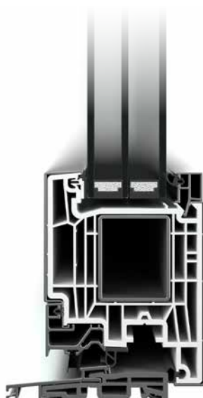
FIN-Door Step Frame – Step Frame 90+2 Aluminium-Aluminium mit Dreifachglas
