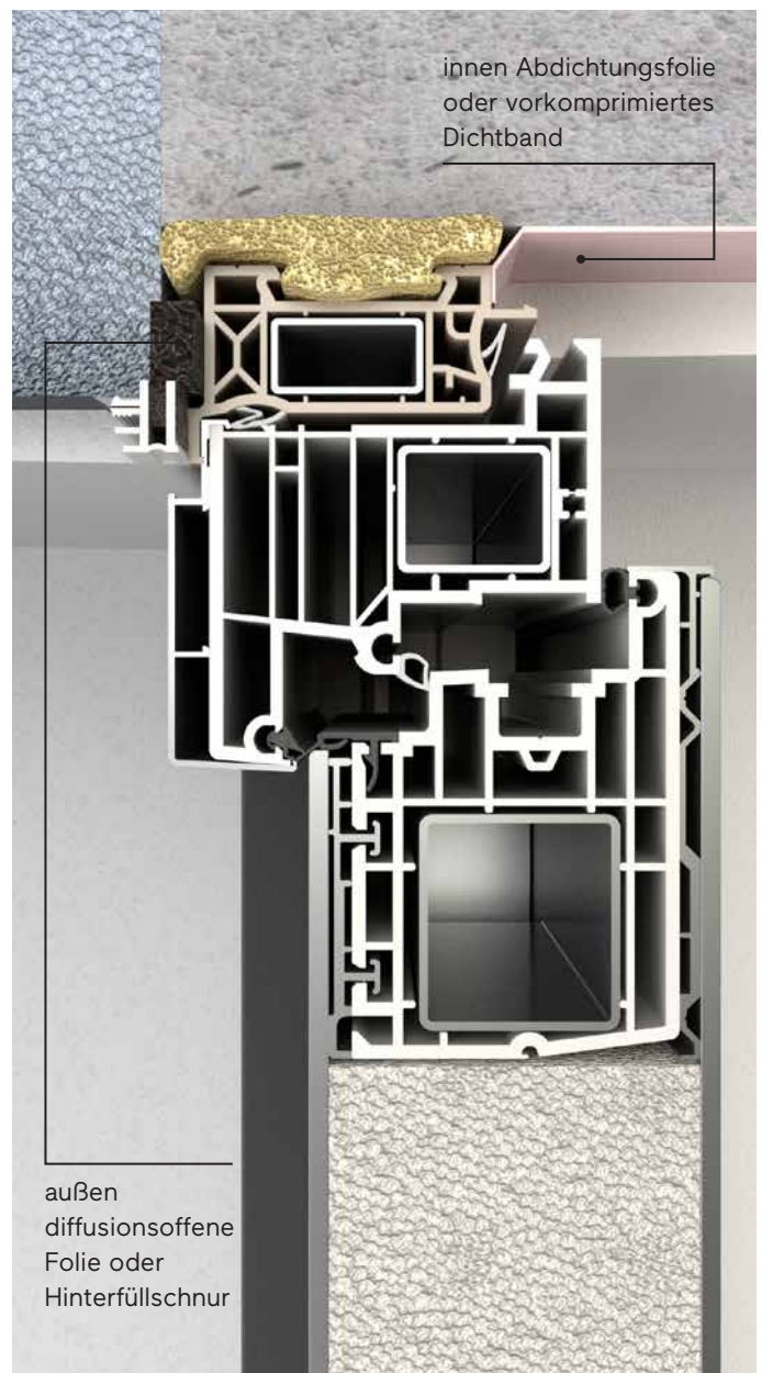
Zweistufige Montage mit Zarge.
