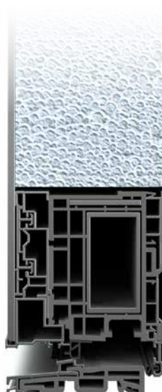
FIN-Door Flat Planar – Step Planar Aluminium-Aluminium mit Türflügel in Aluminium-Aluminium
